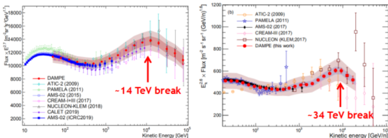
图2. “悟空”号测量得到的40 GeV-100 TeV能段质子宇宙线能谱（左图红点）和70 GeV-80 TeV能段氦核宇宙线能谱（右图红点）。图取自DAMPE collaboration（2019 Sci. Adv.,5, eaax3793；2021 Phys. Rev. Lett., 126, 201102） 研究团队单位：紫金山天文台
