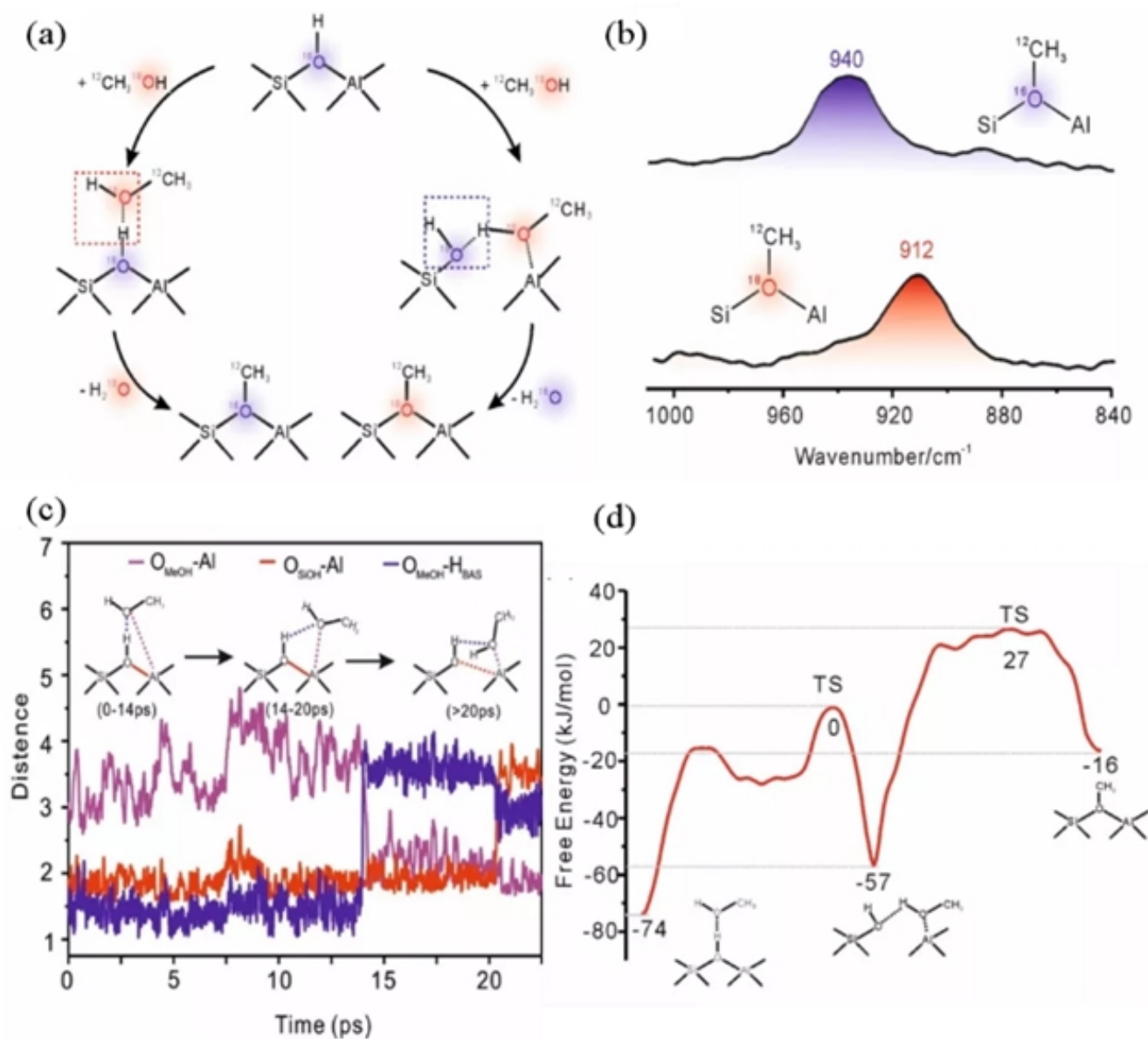
图3：18O-甲醇吸附在SAPO分子筛上的原位漫反射红外实验和从头算分子动力学模拟理论结果。
