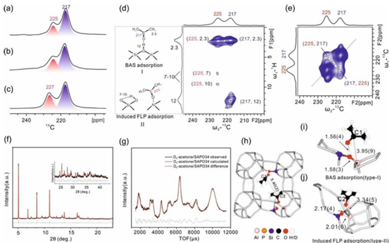
图1：丙酮吸附在SAPO分子筛上的固体核磁实验结果（a-e）；同步辐射X射线衍射/中子衍射实验得到的两种丙酮吸附构型（f-j）。
