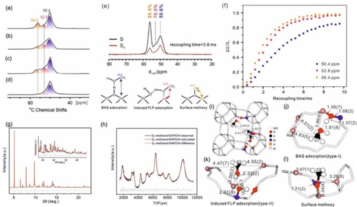
图2：甲醇吸附在SAPO分子筛上的固体核磁实验结果（a-f）和同步辐射X射线衍射/中子衍射实验确定的甲醇吸附构型（g-l）。
