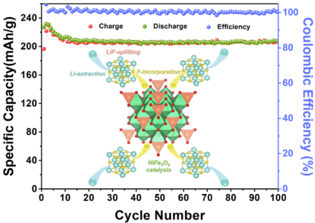
图1.尖晶石结构 \text{NiFe}_2\text{O}_4 催化 \text{LiF} 高效裂解以助力持久高效转换的氟基正极
