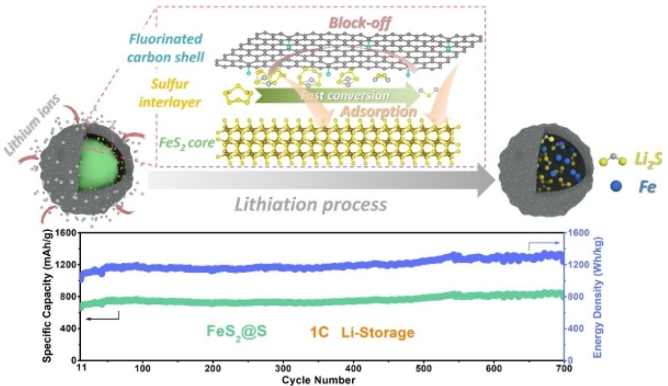
图2.疏硫化表面和亲硫 \text{Fe-S} 结构核心的协同限域/激活效应保证多硫组分的持久高效转换
