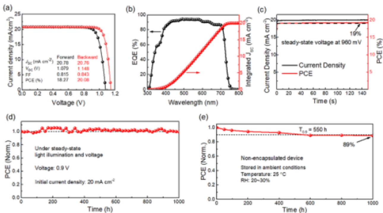
图2.太阳能电池性能表征：（a）最佳电池器件的电流-电压特性曲线；（b）最佳电池器件的外量子效率；（c）最佳电池器件稳态效率测试；（d）最佳电池器件持续工作1000小时稳定性测试；（e）最佳器件（未封装）环境稳定性测试结果
