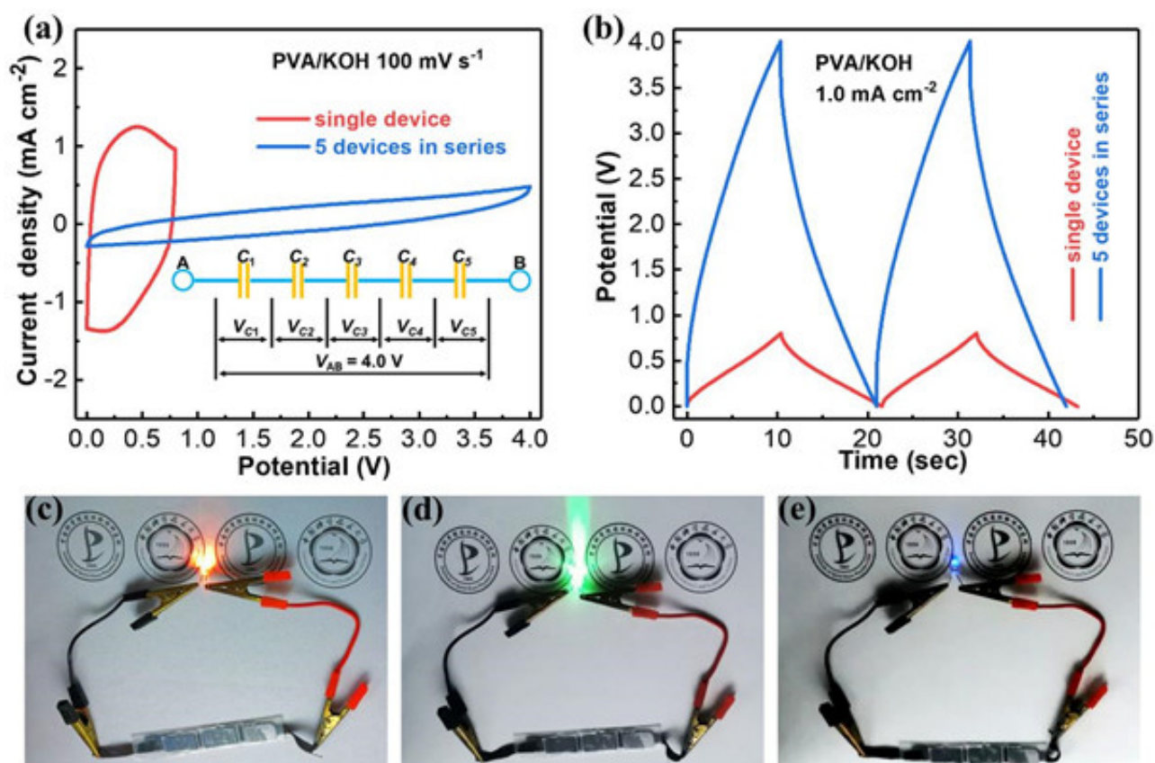
图2.对称固态超级电容器性能测试：(a) 串联器件100 mV s -1 扫速下的电容-电压结果, (b) 串联器件1.0 mA cm -2 电流密度下的充电-放电结果, (c-e) 串联器件驱动不同颜色LED灯实物图
