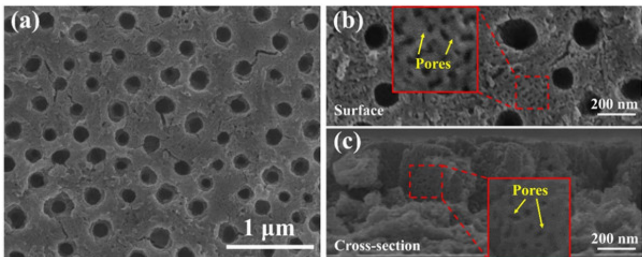
图1.多孔VN薄膜的 (a) 平面低放大倍数扫描电镜结果, (b) 平面高放大倍数扫描电镜结果, (c) 横截面高放大倍数扫描电镜结果图
