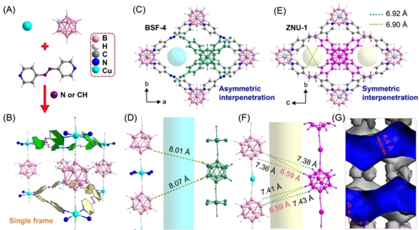
图1：具有相近网络结构、不同穿插对称性的BSF-4和ZNU-1的比较
