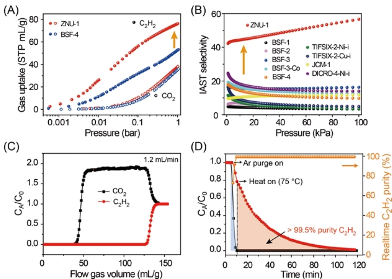
图2：(A) ZNU-1和BSF-4在298K条件下的乙炔和二氧化碳吸附等温线；(B) 性能最佳的阴离子杂化MOFs对1：1的C 2 H 2 /CO 2 混合物的IAST吸附选择性比较；(C) ZNU-1在298 K下C 2 H 2 /CO 2 （50/50）的穿透曲线；(D) Ar吹扫下ZNU-1的解吸曲线
