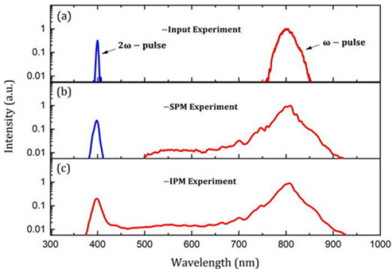
图2.紫外增强型超连续光谱
