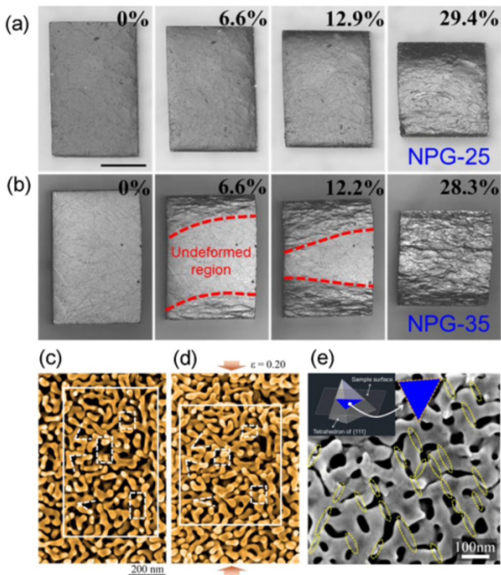
图2.纳米多孔金的均匀与非均匀变形。相对密度为0.27的NPG-25样品。(a)和相对密度为0.36的NPG-35样品；(b)压缩不同应变后的表面形貌光镜照片；(c-d)为NPG-25样品压缩20%前后局部变形情况，可见孔棱发生弯曲变形和悬挂孔棱发生搭接；(e)压缩10%的NPG-35中，变形带内的孔棱发生位错雪崩式滑移变形的痕迹
