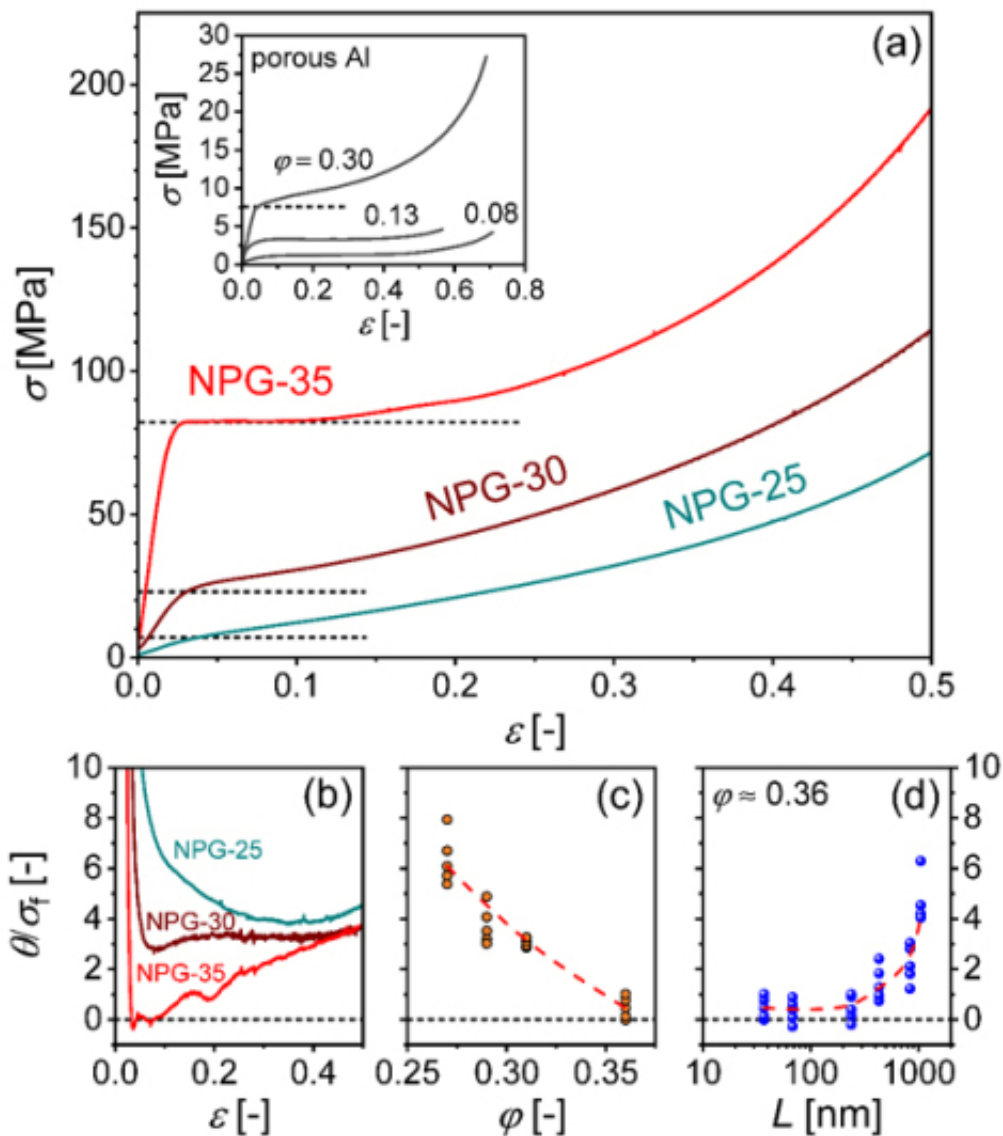
图1.纳米多孔金的压缩变形行为。(a)不同相对密度纳米多孔金的压缩应力应变曲线，小图为不同相对密度常规多孔铝的压缩应力应变曲线；(b)不同相对密度纳米多孔金归一化后的加工硬化率随压缩应变的变化情况；(c)纳米多孔金归一化加工硬化率随相对密度的变化；(d)相对密度为0.36的NPG-35样品的加工硬化率随孔棱尺寸的变化情况
