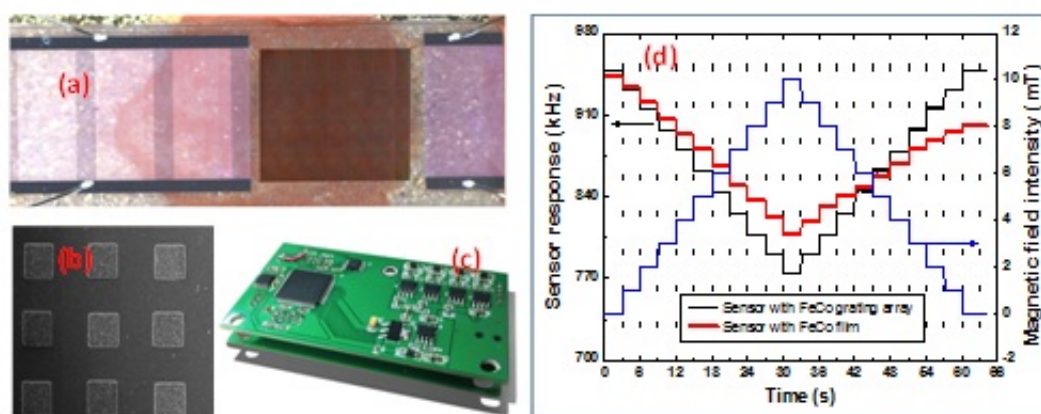
新型声表面波电流传感器 (a) 传感器件, (b) 图形化磁敏薄膜, (c) 传感器原型样机, (d)
