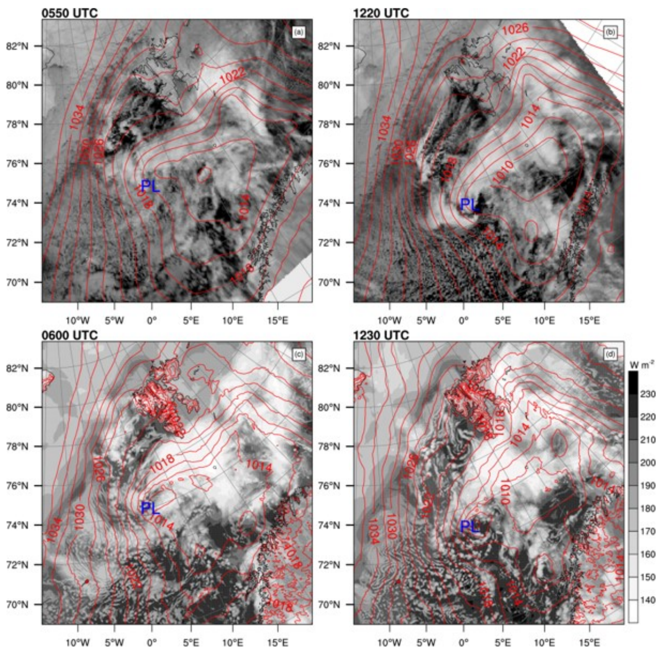
个例模拟，(a) (b) ERA-Interim 海平面气压和AVHRR卫星图像，(c) (d) 模式的海平面气压和OLR结果 研究团队单位：大气物理研究所
