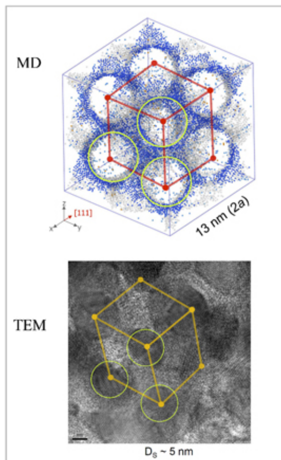
图2.Schwarz-D受限晶体热稳定性尺寸效应、晶体受限效应、分子动力学模拟及实验观测对照
