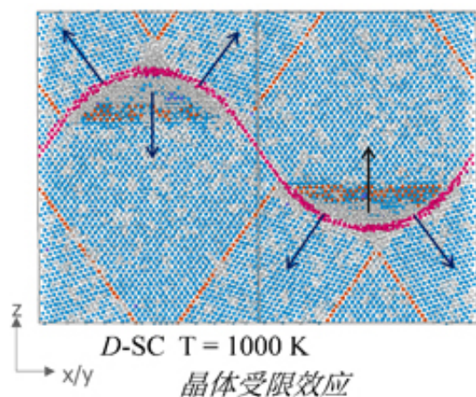
图2.Schwarz-D受限晶体热稳定性尺寸效应、晶体受限效应、分子动力学模拟及实验观测对照
