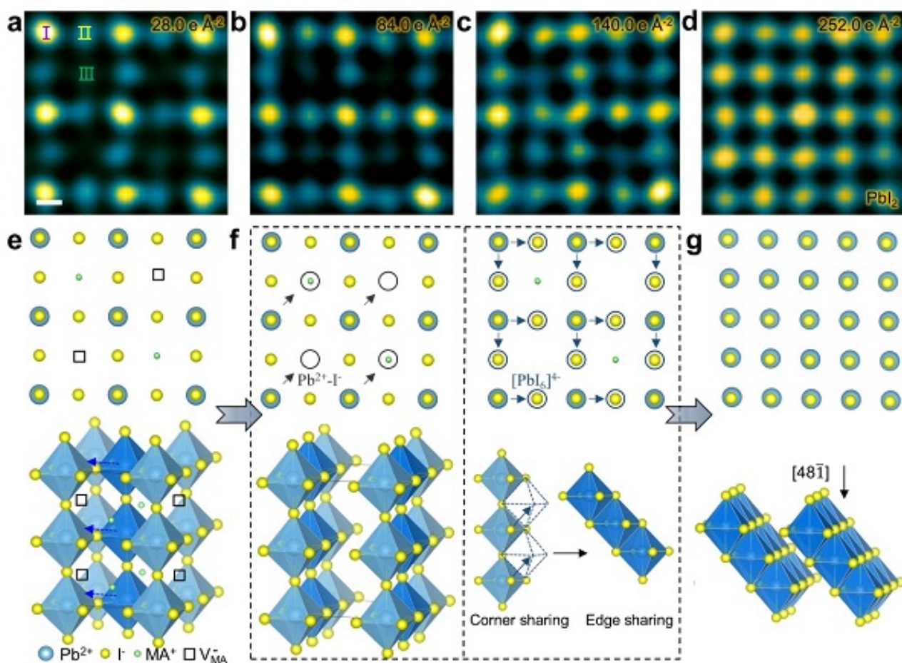
MAPbI 3 原子尺度降解路径
