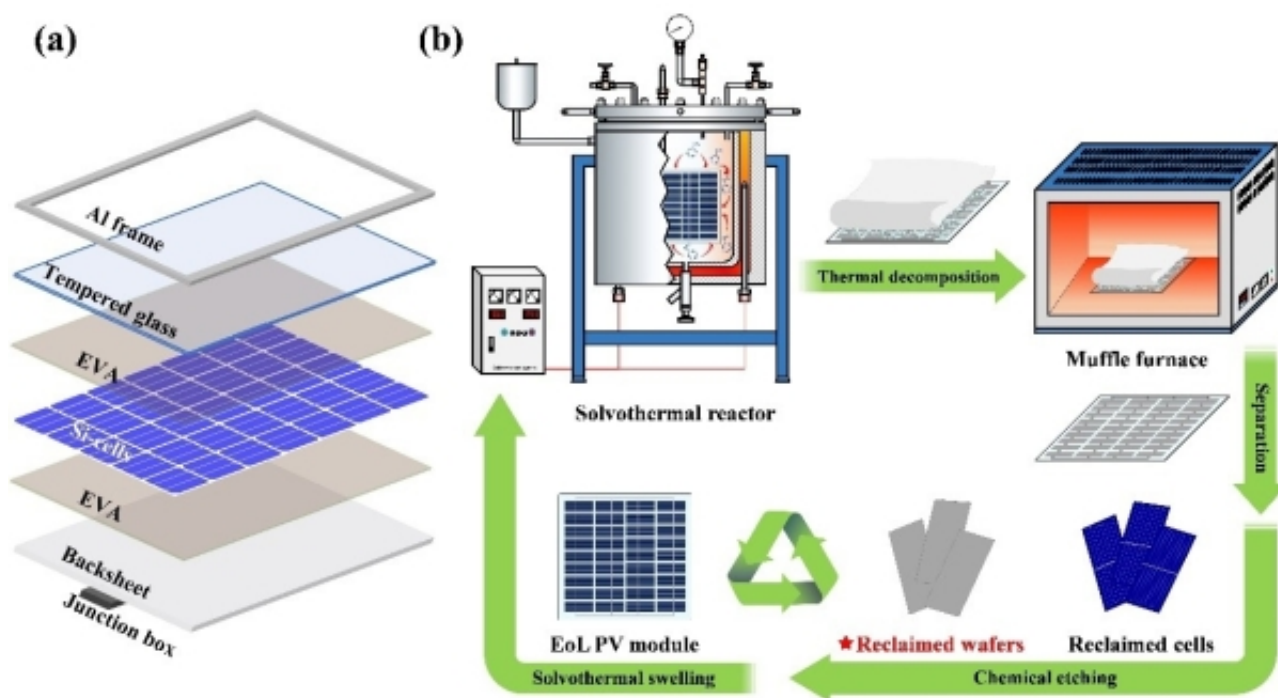
晶体硅光伏组件结构示意和资源回收工艺流程
