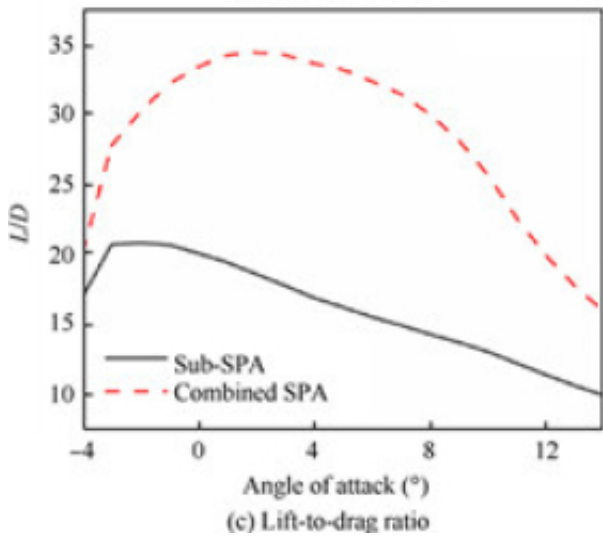
图3.组合式太阳能无人机气动性能分析
