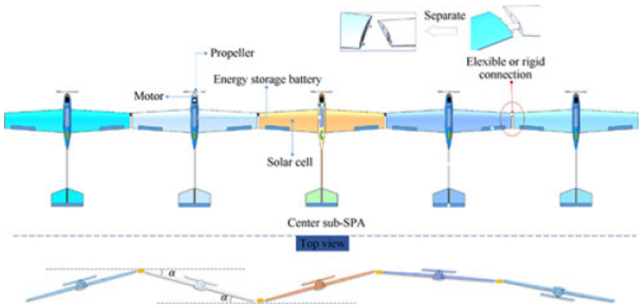
图1.组合式无人机的基本形式
