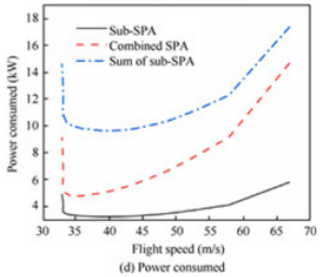
图3.组合式太阳能无人机气动性能分析
