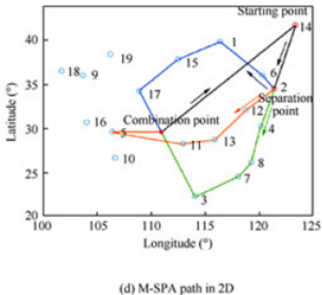
图4.组合式太阳能无人机路径规划
