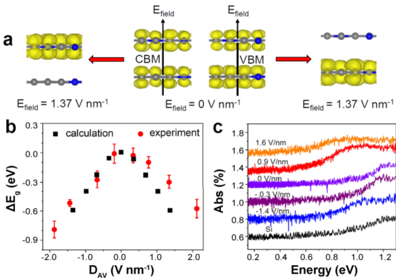
图3 双层 C_3N 在电场下的带隙调制
