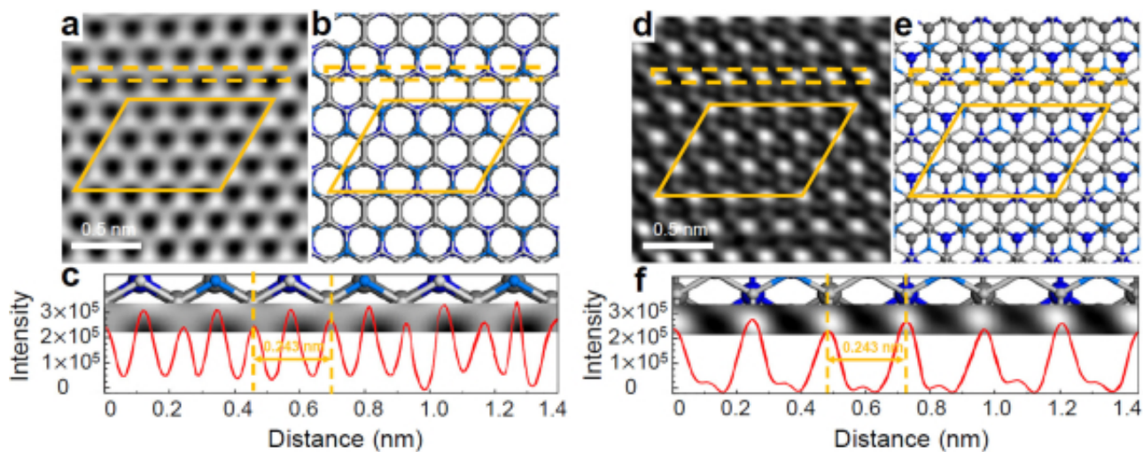
图2 AA (a-c) 及AB (d-f) 堆垛双层 C_3N 的HAADF-STEM图像
