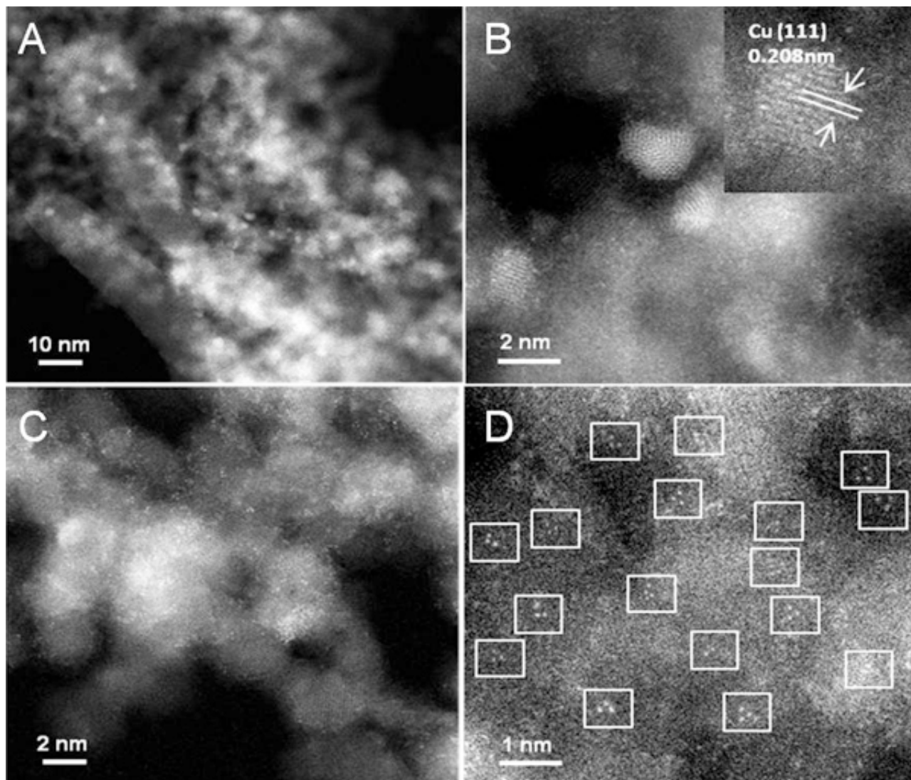
图1.A、B：Cu 3 金属团簇（Cu 3 /ND@G）的球差电镜表征；C、D：亚纳米尺度Cu 3 金属团簇（Cu 3 /ND@G）的球差电镜表征
