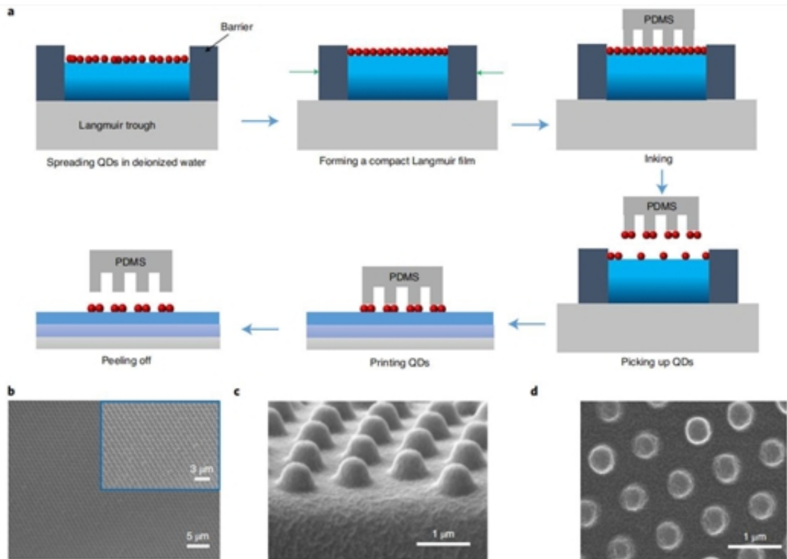
(a) LB-TP工艺示意图；(b) 微结构PDMS印章的光学显微镜图像；(c-d) 微结构PDMS印章的扫描电子显微镜图像（直径，间距和高度均为500 nm）。福州大学供图
