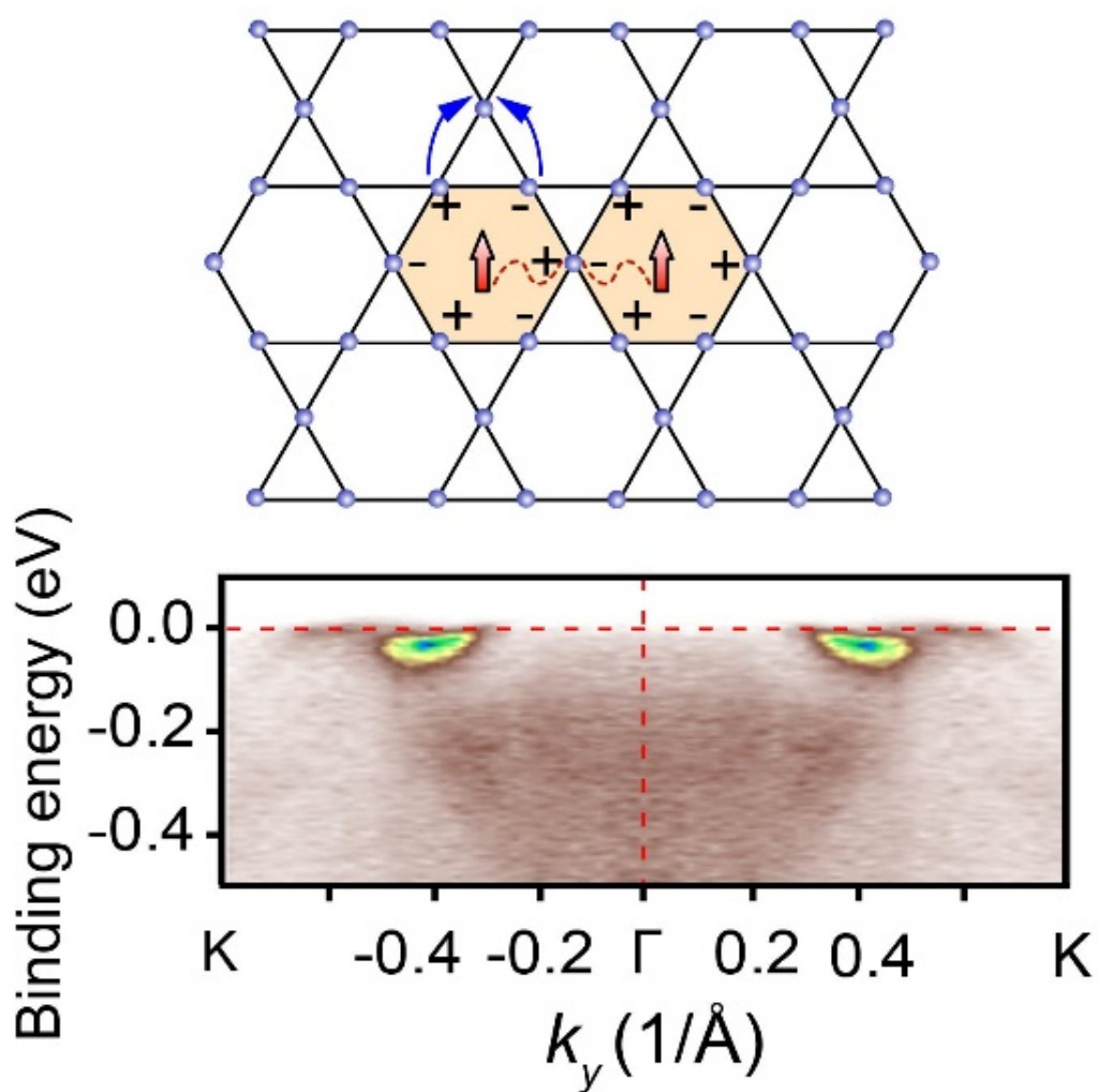
kagome晶格上电子态相消干涉导致局域化和自旋耦合导致铁磁性的示意图(上图);角分辨光电子能谱实验观测下的平带(下图)
