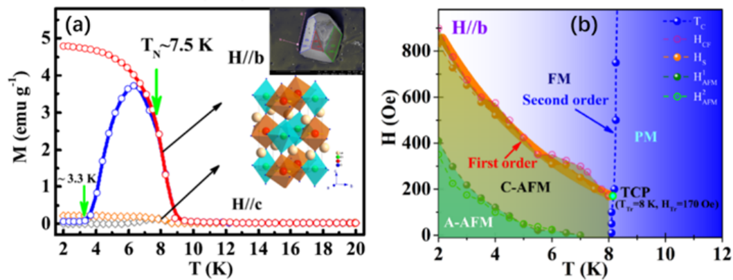
图:(a)La 2 ZnIrO 6 的晶体结构、单晶形貌和不同方向的磁化强度;(b)H-T相图以及三重临界点行为
