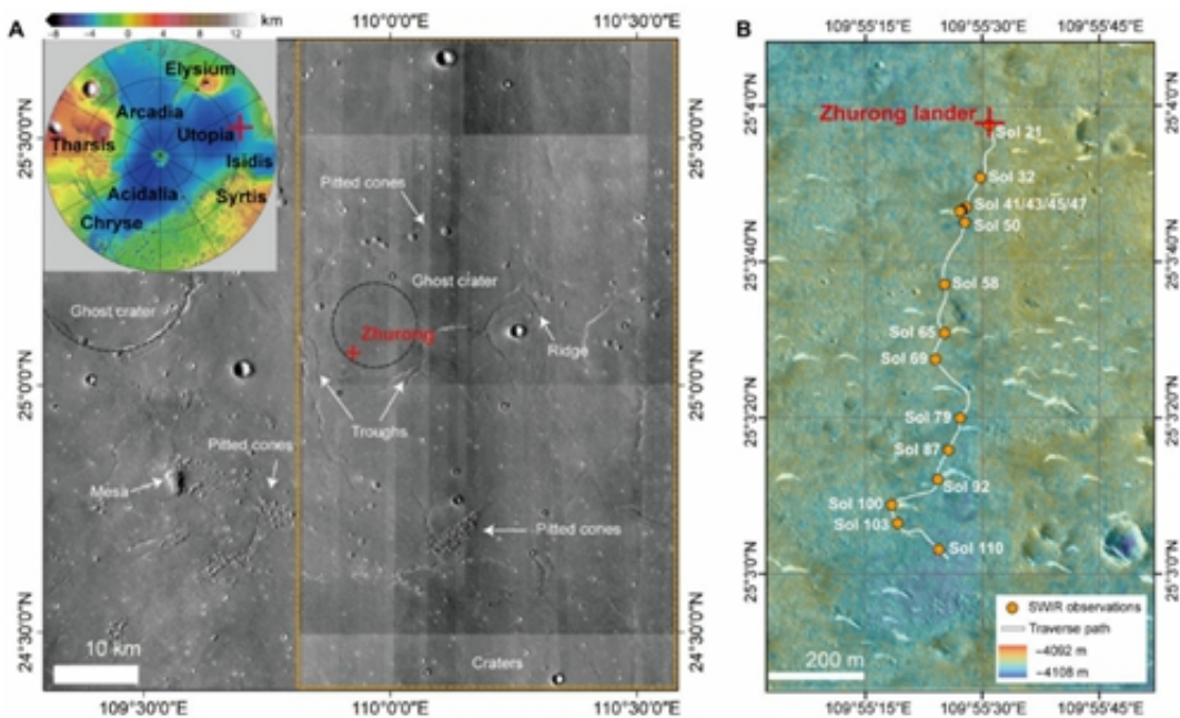
图1. (A) “祝融号”着陆点地貌图。(B) “祝融号”巡视路线图。
