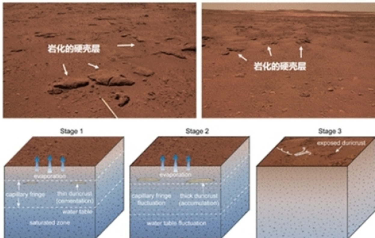
图3.祝融着陆区富含硫酸盐的岩化硬壳形成过程示意图。第1阶段：蒸发发生在地下水位附近和
