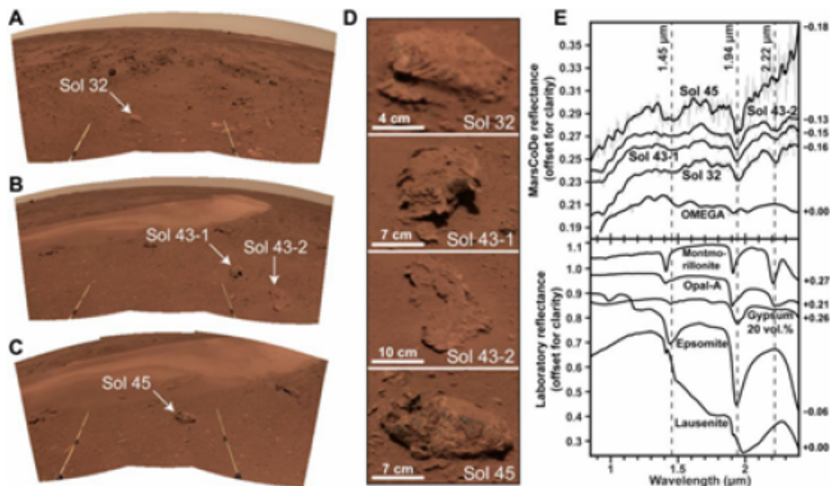
图2.导航相机全景图 ( A ) sol 32、 ( B ) sol 43和 ( C ) sol 45。白色箭头指示短波红外光谱观测目标岩石的位置。( D ) 光谱测量岩石的放大图像。( E ) 短波红外光谱与实验室光谱的比较。上图显示平滑的短波红外光谱 ( 粗实线 ) 叠加在原始光谱 ( 细实线 )。
