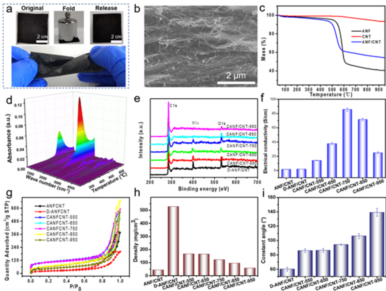
图3.碳纳米管气凝胶薄膜的结构与性能
