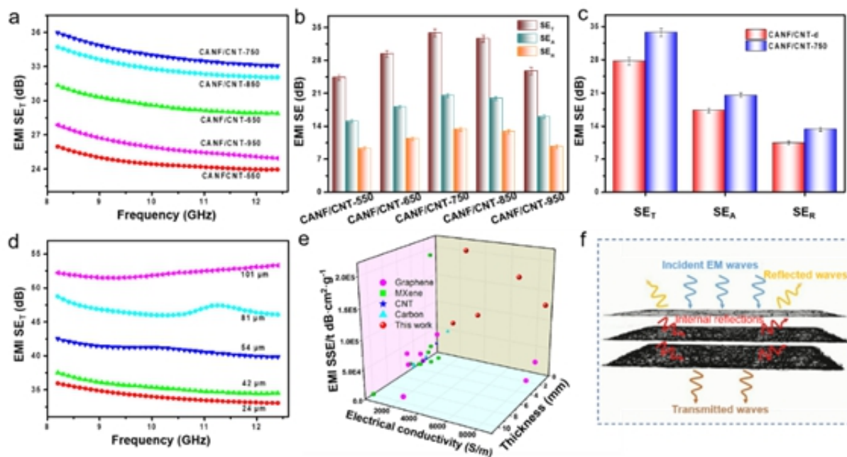
图4.碳纳米管气凝胶薄膜的电磁屏蔽性能
