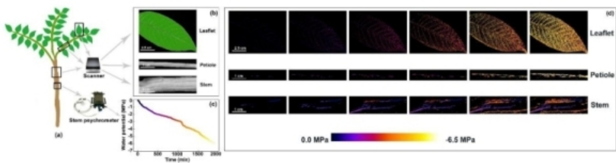
图1.利用可视化技术对复叶树种枝条不同部位的栓塞发生动态过程进行连续测定
