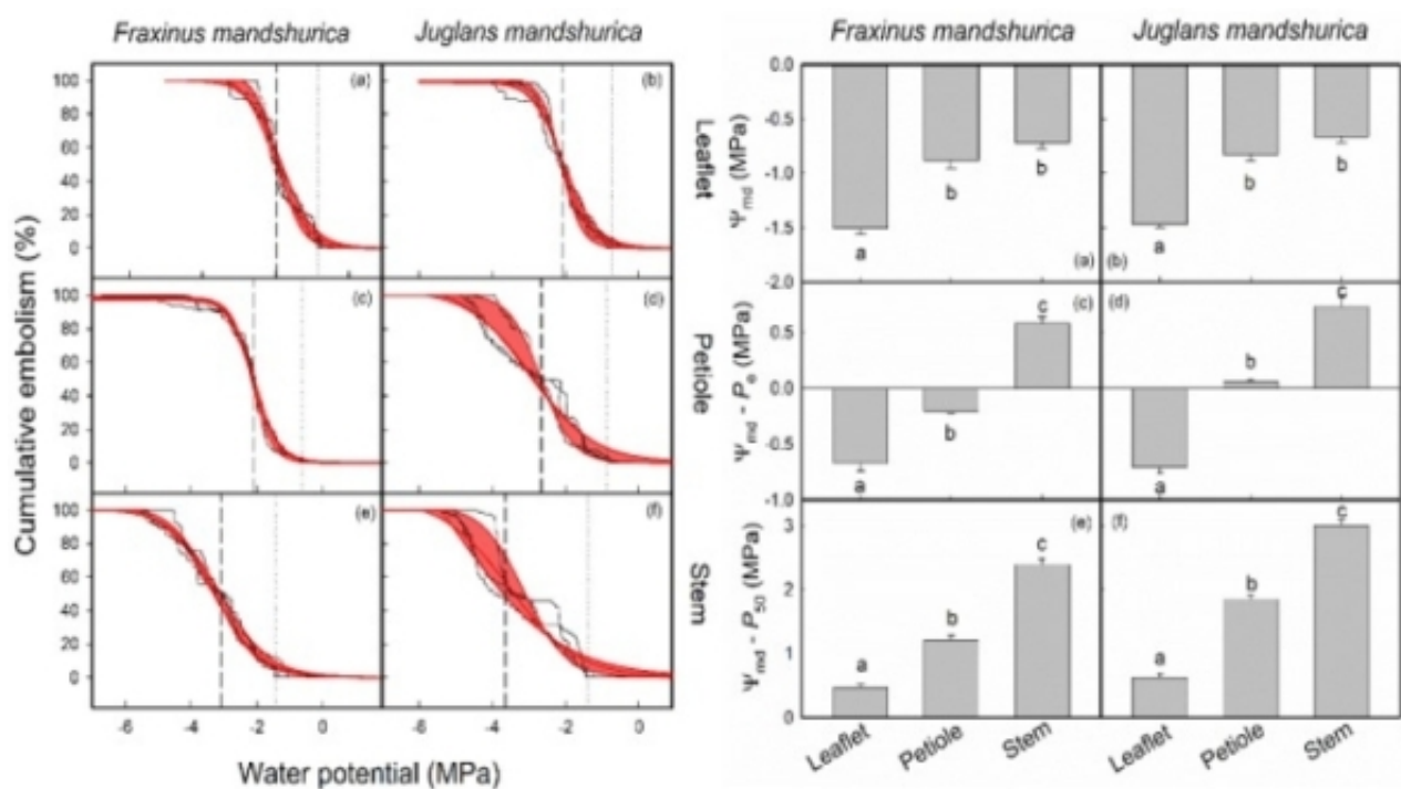
图2.叶片、叶柄和茎的木质部脆弱性曲线（左）和正午水势及水力安全边界（右） 研究团队单位：沈阳应用生态研究所
