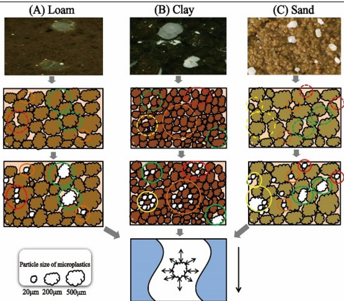
图2.微塑料颗粒影响土壤水力特征的潜在作用机制
