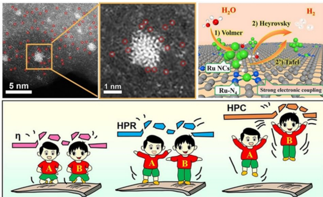
氮掺杂介孔碳负载Ru单原子和纳米团簇催化剂NMC-Ru SA+NC 研究团队单位：青岛生物能源与过程研究所
