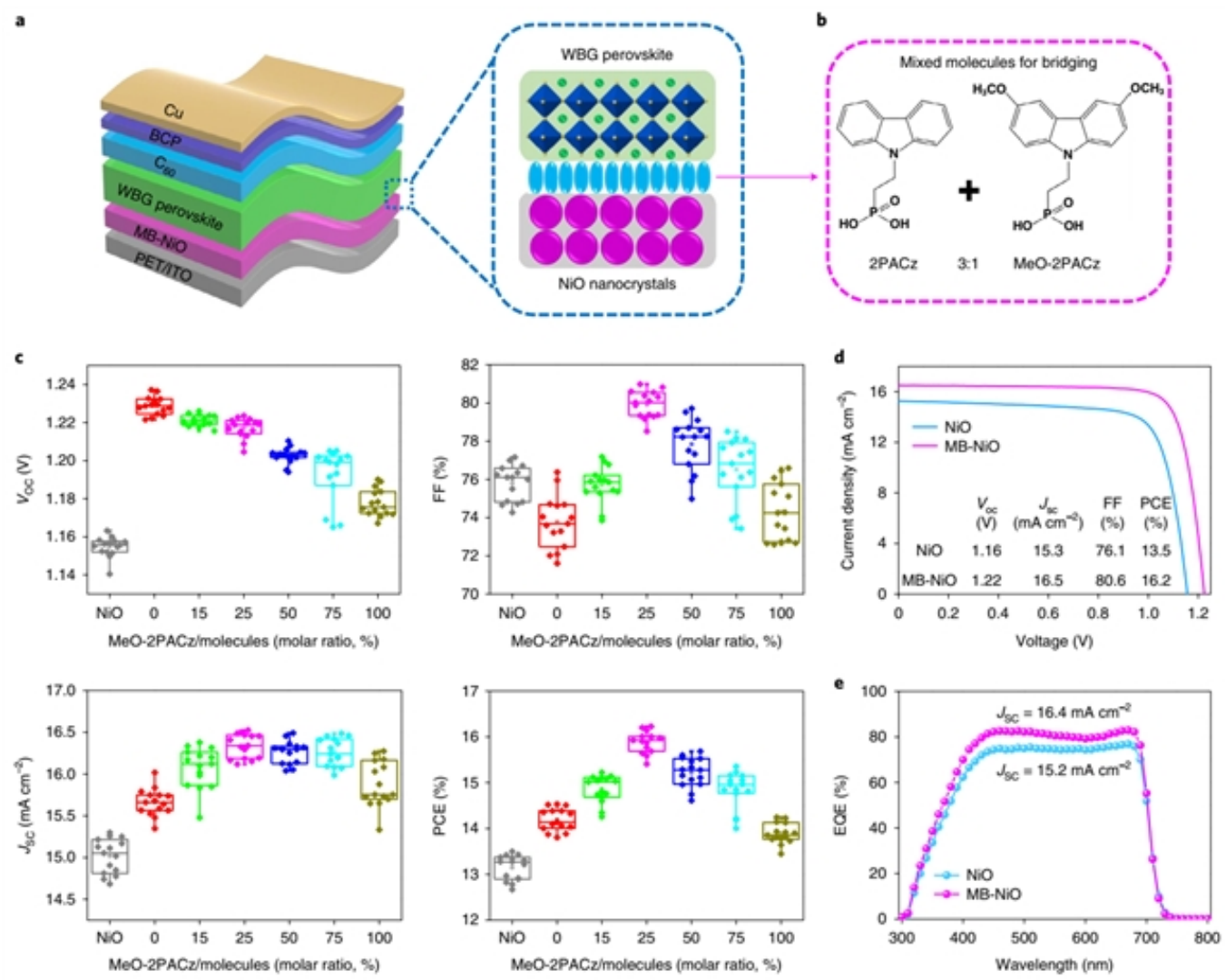
图1：柔性宽带隙钙钛矿太阳电池的器件结构及光伏性能。
