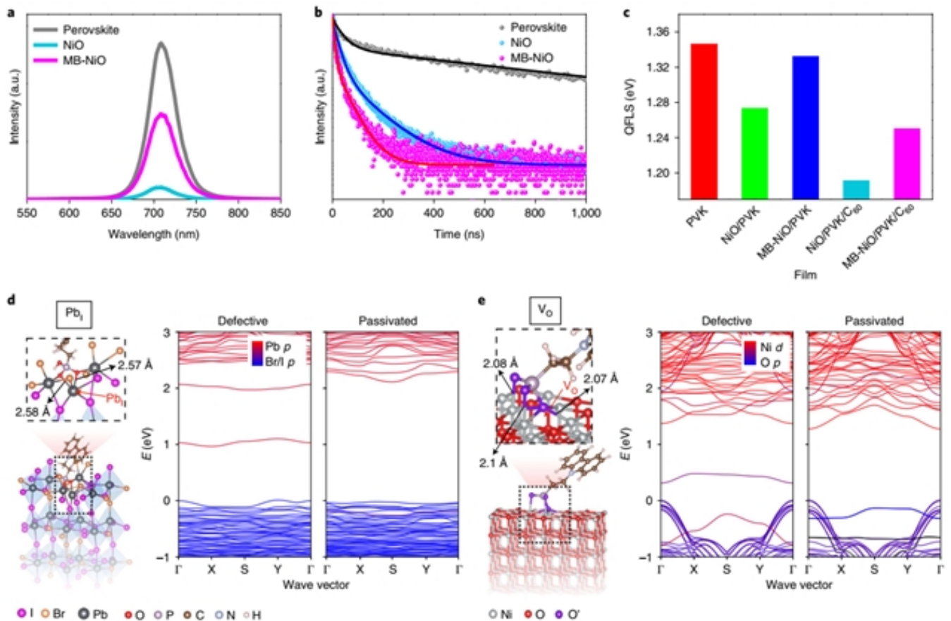
图3：（a-c）基于不同空穴传输层的宽带隙钙钛矿薄膜的载流子动力学表征；（d，e）桥接分子（2PACz）钝化钙钛矿与氧化镍表面缺陷的第一性原理模拟。
