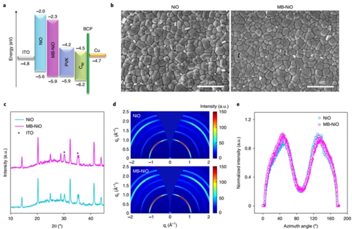
图2：宽带隙钙钛矿薄膜材料表征。
