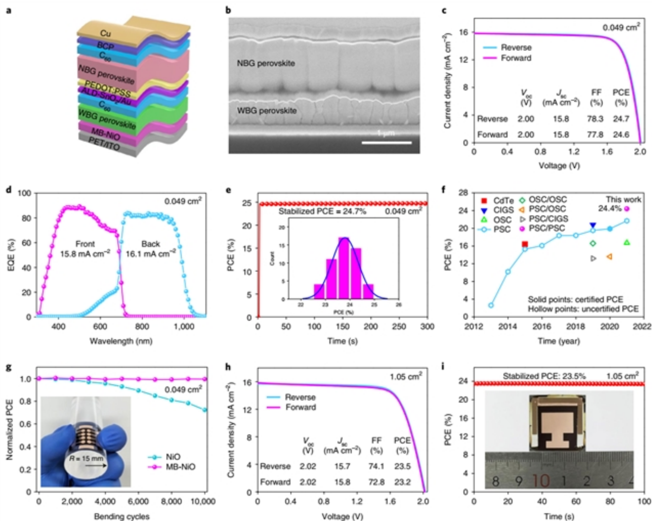
图4：柔性全钙钛矿叠层太阳电池的光伏性能和弯曲耐折度表征。
