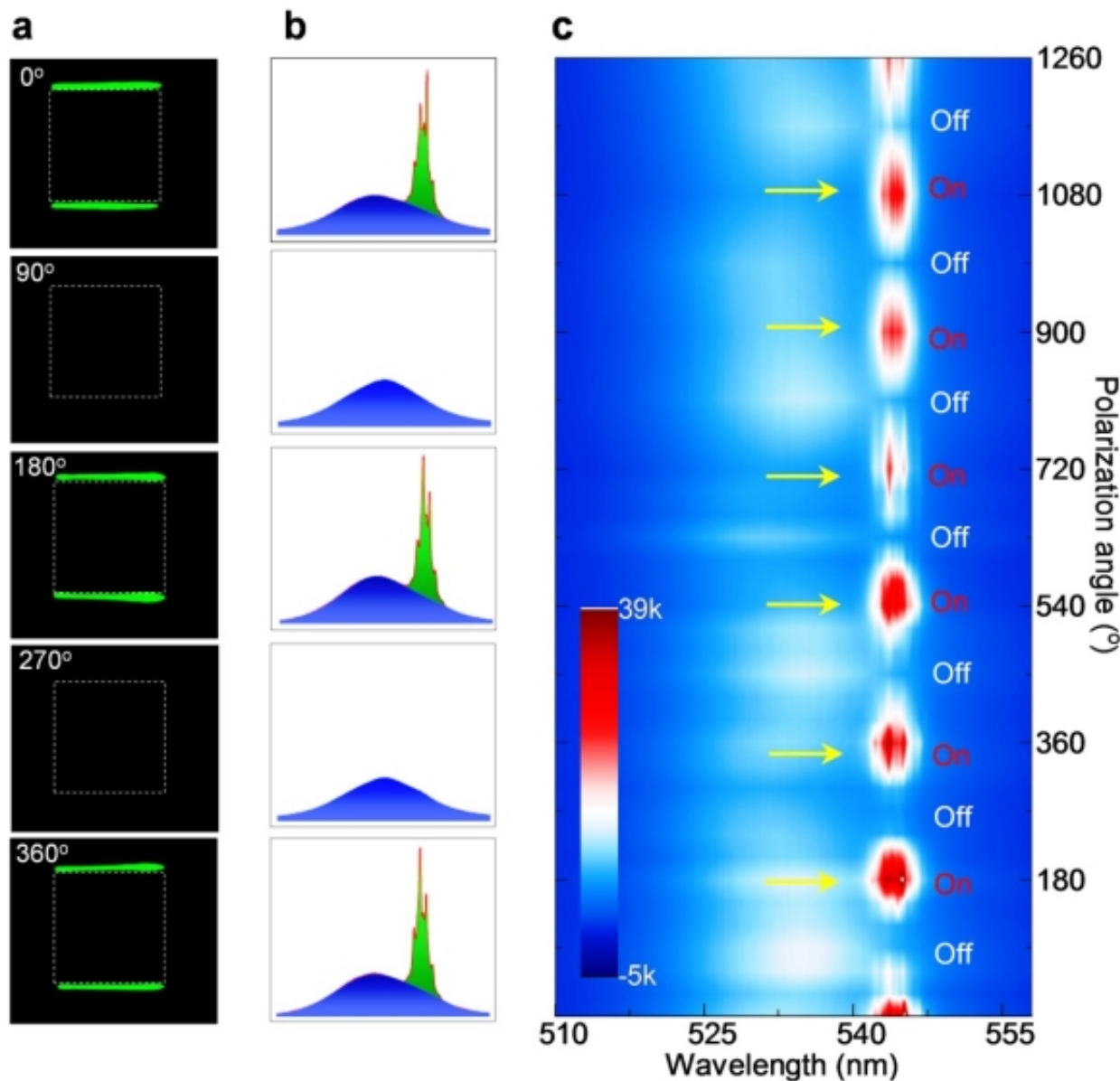
图3 不同偏振角度下的荧光成像(a)和光谱(b)；(c)通过偏振实现激光ON/OFF调制。 研究团队单位：国家纳米科学中心
