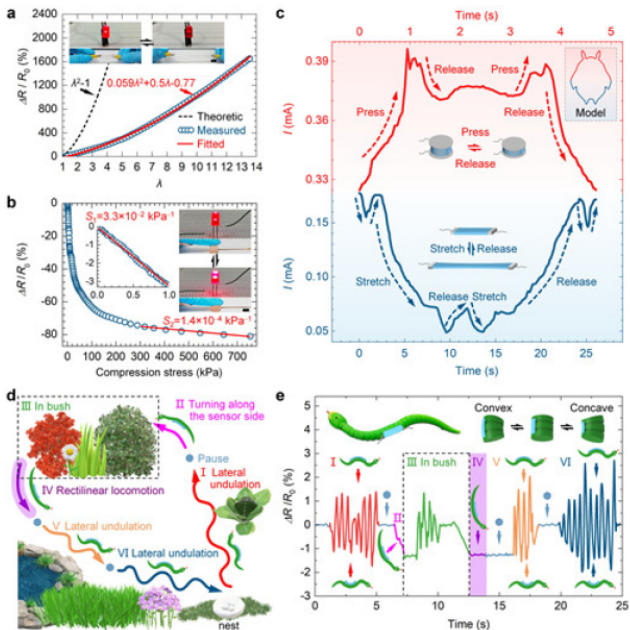
图3.类皮肤水凝胶传感器的感知性能调控
