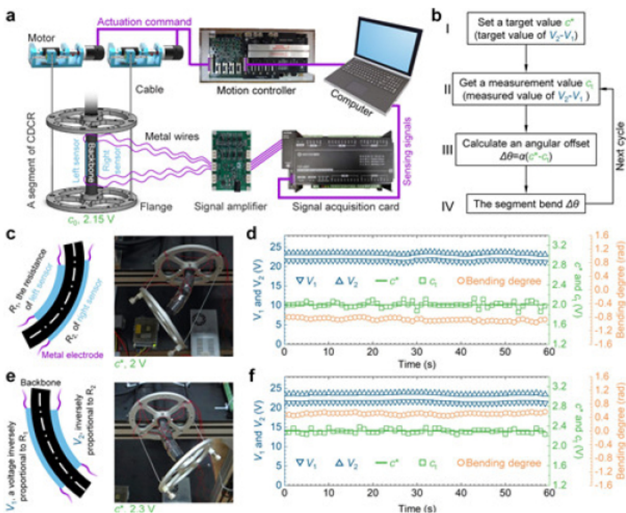
图5.绳驱动连续体机器人水凝胶传感器感知系统的闭环控制
