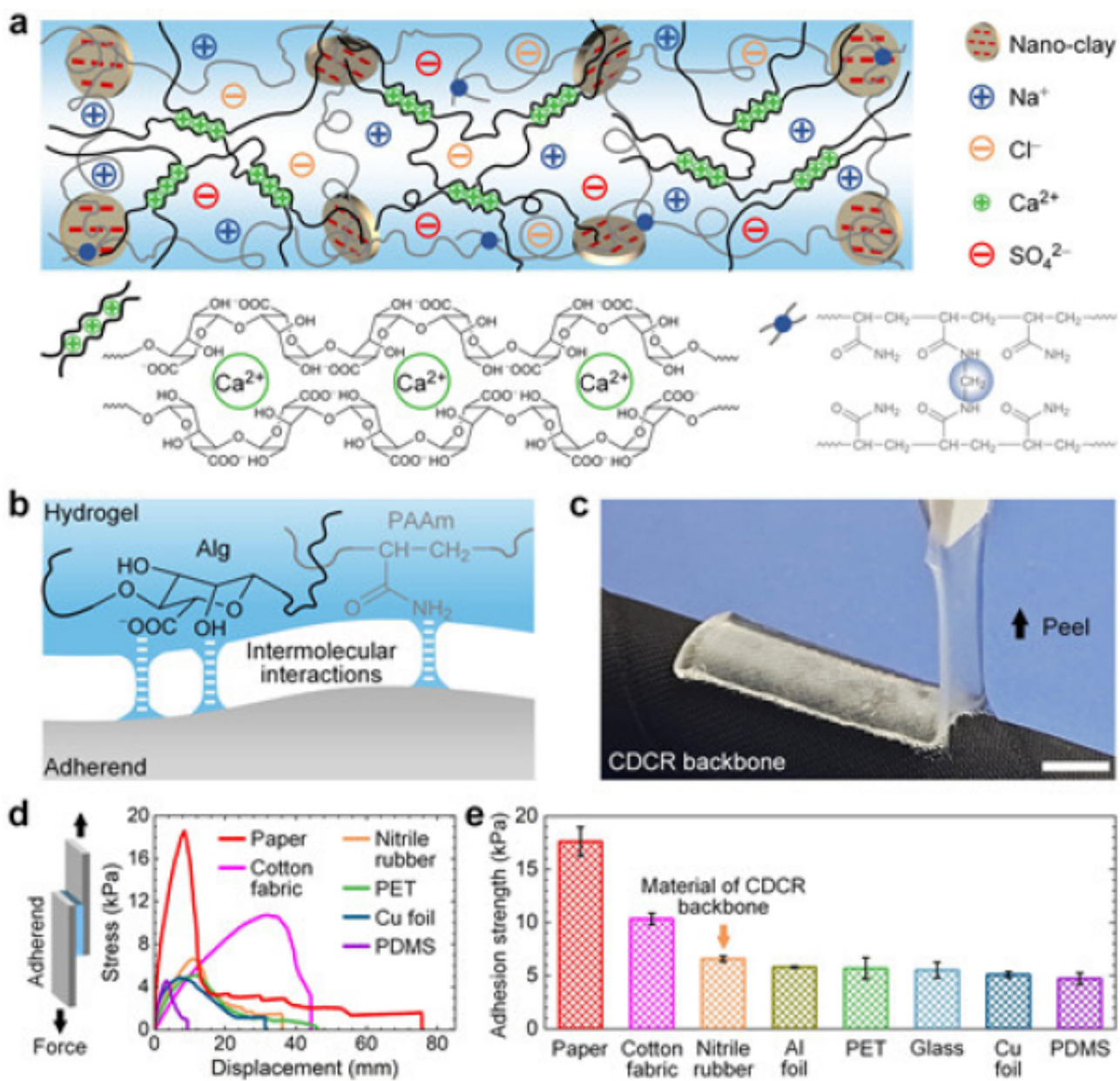
图2.类皮肤水凝胶传感器的构建、修复与黏附等性能调控
