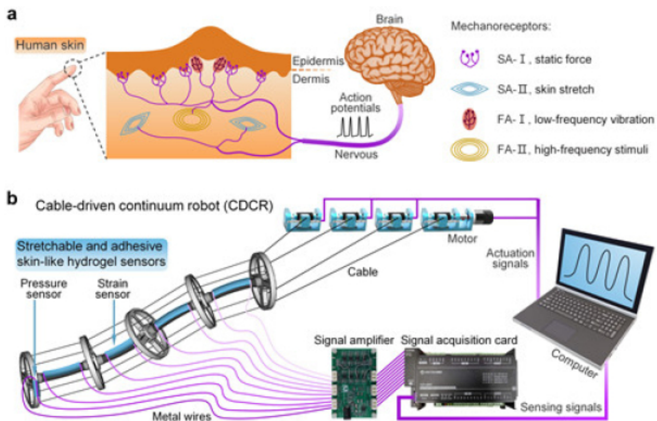
图1.类皮肤水凝胶传感器用于绳驱动连续体机器人的感知
