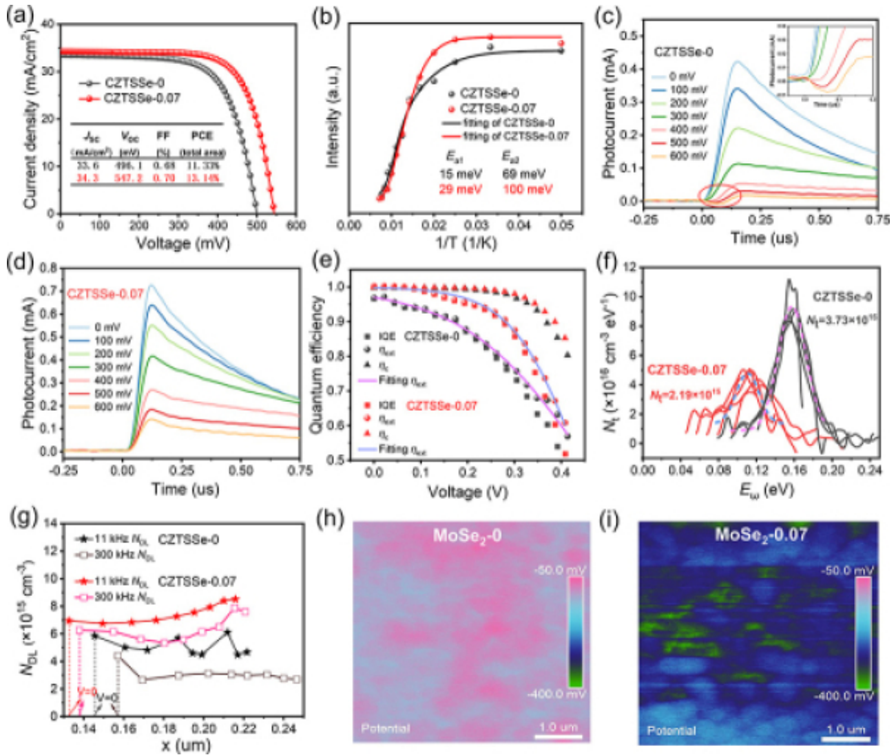
图2 (a) 基于CZTSSe-0-GeO 2 和CZTSSe-0.07-GeO 2 电池J-V曲线；CZTSSe-0-GeO 2 和CZTSSe-0.07-GeO 2 器件的缺陷及复合性质；(b)由稳态荧光谱得到的激活能 E_a ；(c)CZTSSe-0-GeO 2 样品的变偏压TPC；(d) CZTSSe-0.07-GeO 2 样品的变偏压TPC；(e) 基于TPC和TPV测试获得的收集效率 \eta_c 和抽取效率 \eta_{ext} ；(f) 基于导纳谱获得的缺陷态密度；(g) 基于DLCP表征获得载流子密度；(h) MoSe 2 -0-GeO 2 样品表面电势；(i) MoSe 2 -0.07-GeO 2 样品表面电势。
