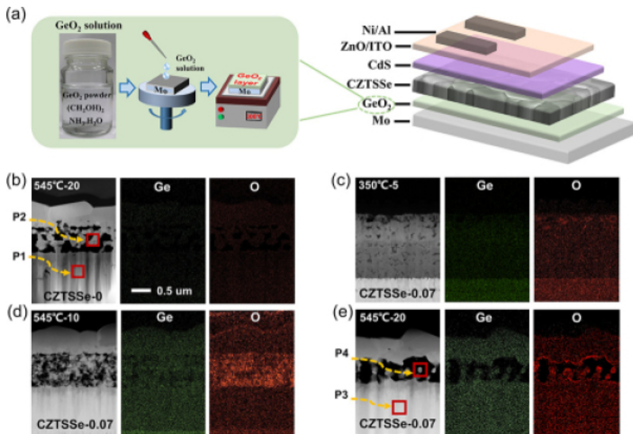
图1 (a) 旋涂法制备 \text{GeO}_2 层及CZTSSe器件结构示意图；CZTSSe-0- \text{GeO}_2 和CZTSSe-0.07- \text{GeO}_2 薄膜中Ge和O元素在不同硒化条件下的STEM-EDS扫描图：(b) CZTSSe-0- \text{GeO}_2 薄膜在545°C-20，(c) CZTSSe-0.07- \text{GeO}_2 薄膜在350°C-5，(d) CZTSSe-0.07- \text{GeO}_2 薄膜在545°C-10，(e) CZTSSe-0.07- \text{GeO}_2 薄膜在545°C-20。
