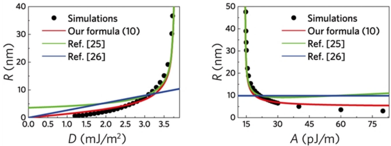
图2：本文解析结果与数值模拟和原有理论的对比
