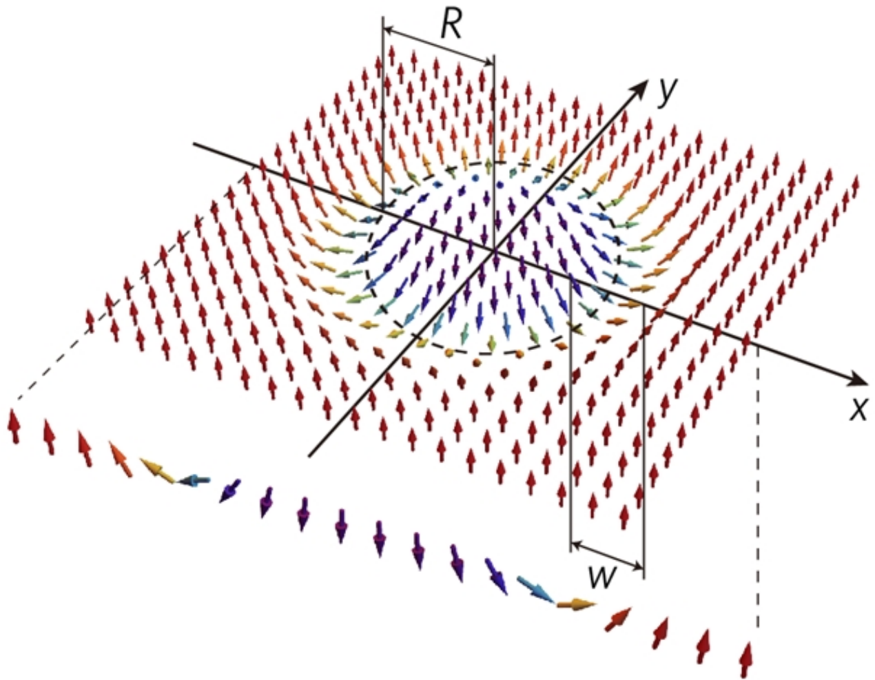
图1：斯格明子(skyrmion)的结构及其与360°磁畴壁结构的对应
