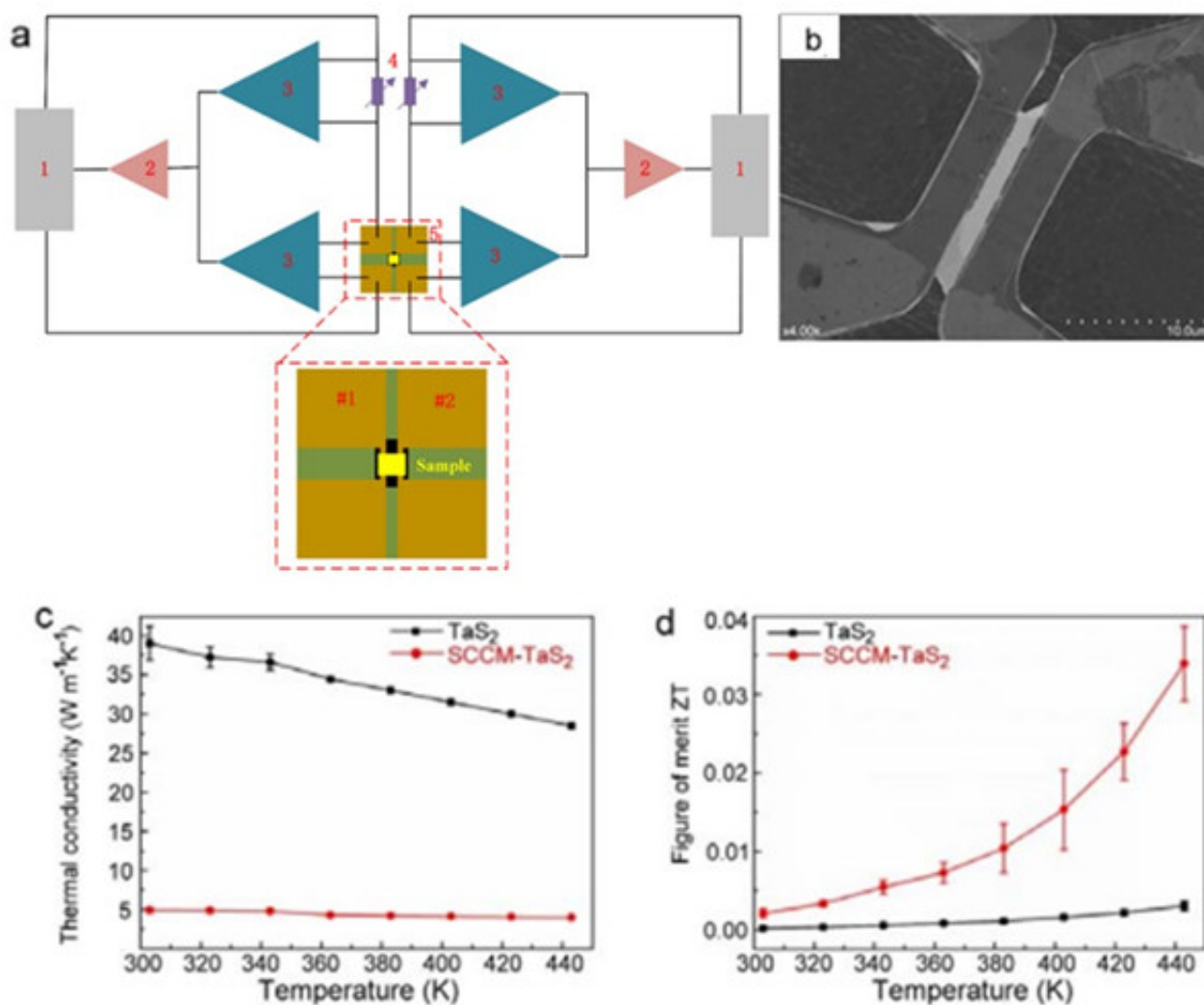
图2.TaS 2
