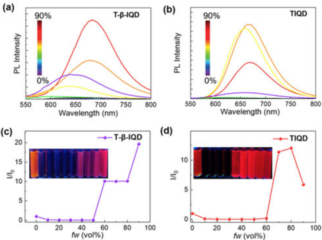
图3.分子的AIE效应特征
