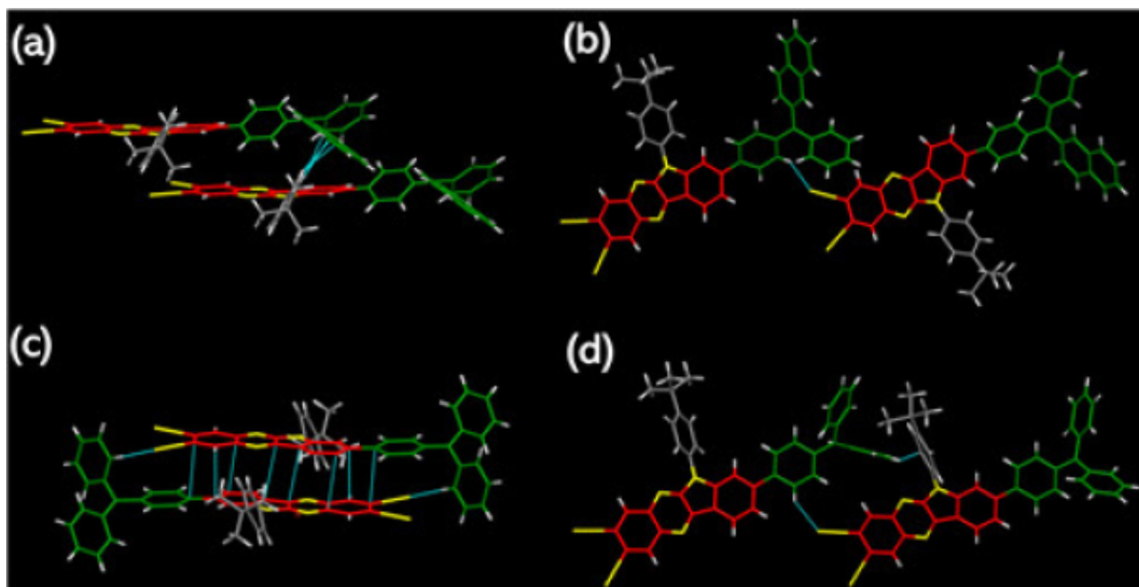
图1.分子内-分子间弱相互作用
