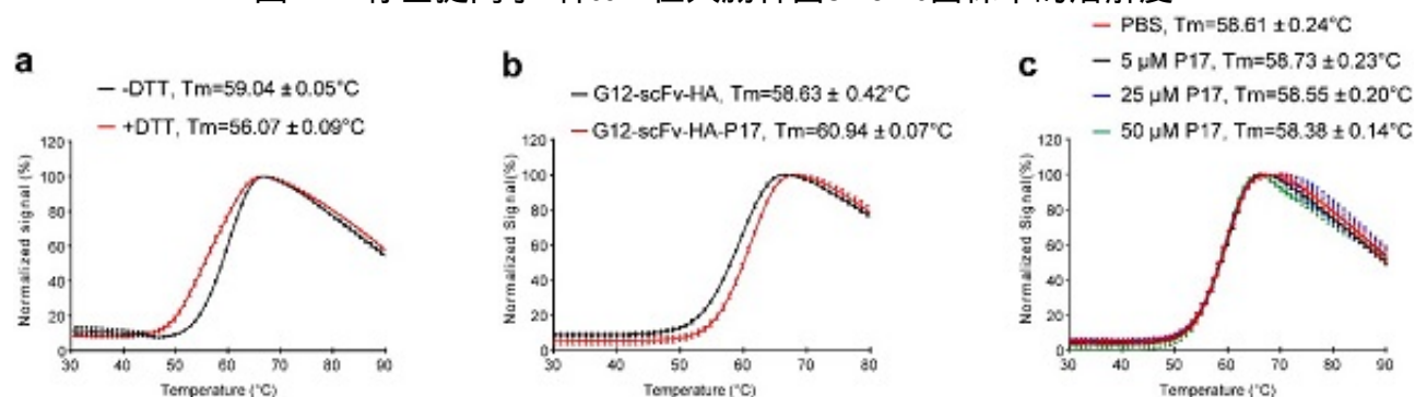
图2.P17标签提高了G12-scFv的热稳定性
