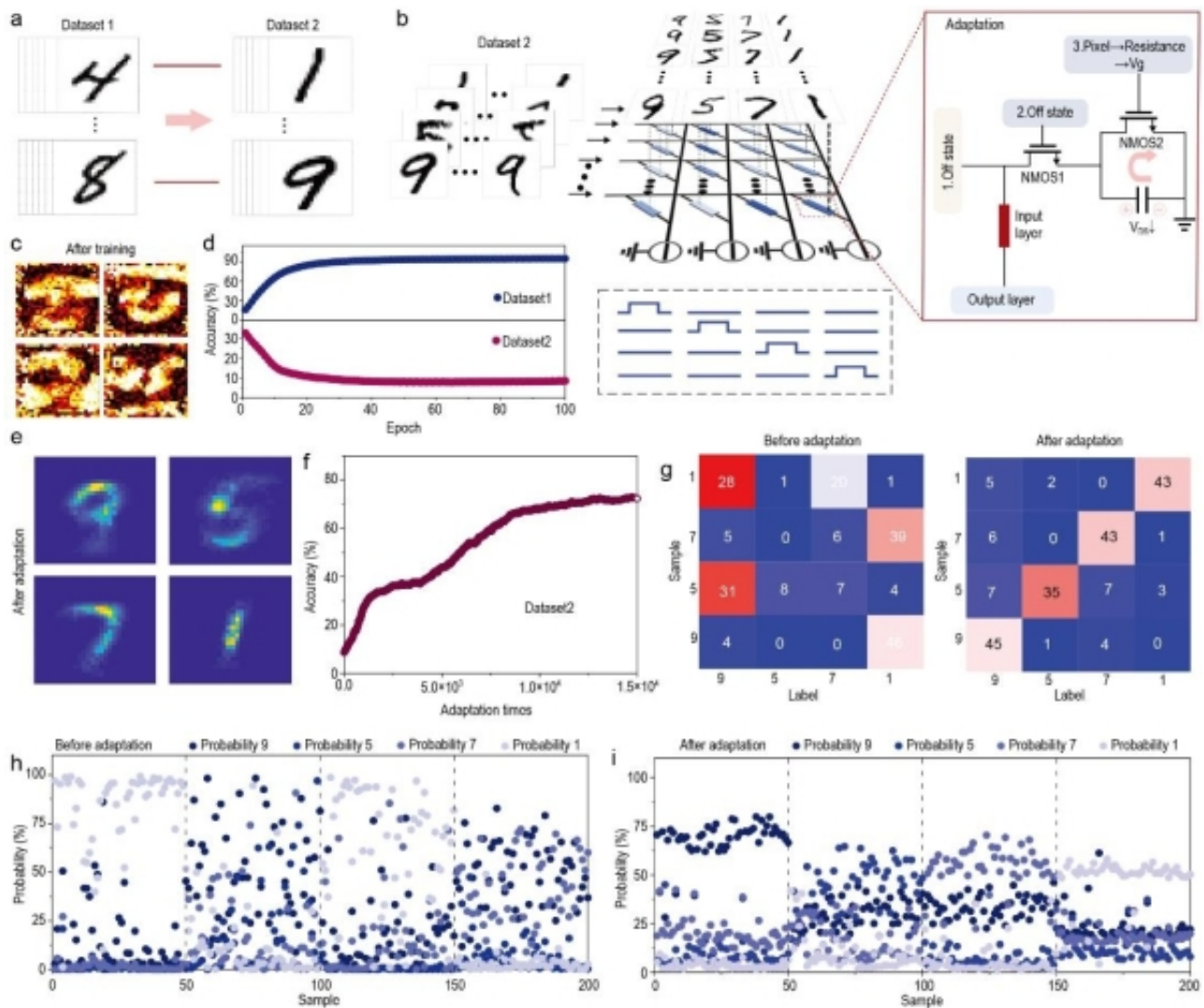
图3.数字识别的自适应仿真。a、Dataset1和dataset2，b、人工神经网络的权重映射图像，c、dataset1和dataset2的识别精度，d、人工神经网络权重的自适应调整，e、自适应后权重映射图像，f、识别精度与映射图像数量的关系，g、适应前后的分类识别，h-i、每个样本的概率。研究团队单位：半导体研究所
