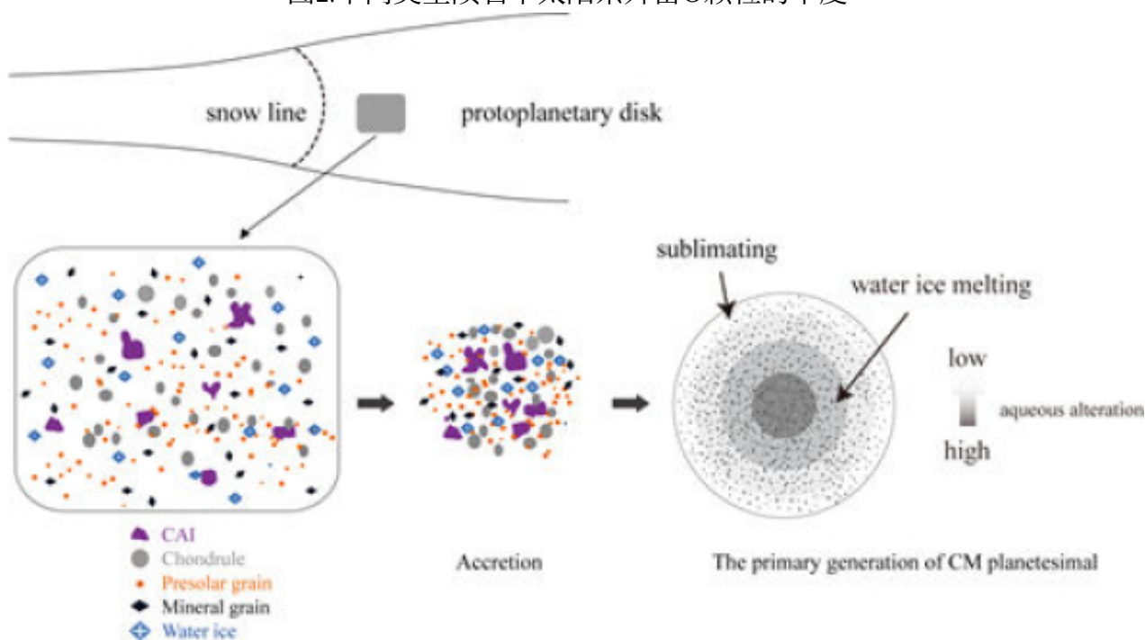
图3.CM型碳质小行星演化示意图 研究团队单位：国家空间科学中心
