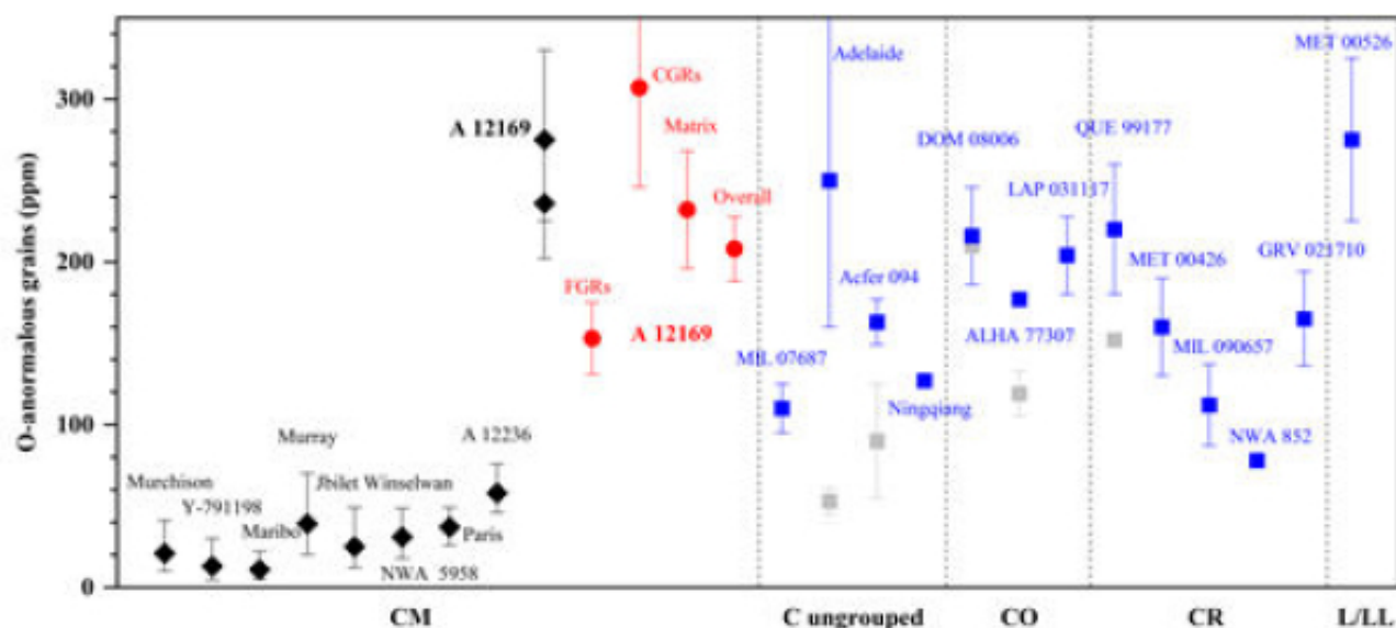
图2.不同类型陨石中太阳系外富O颗粒的丰度
