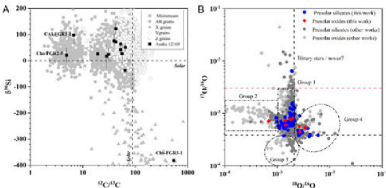
图1.A、太阳系外富碳颗粒，B、太阳系外富氧颗粒
