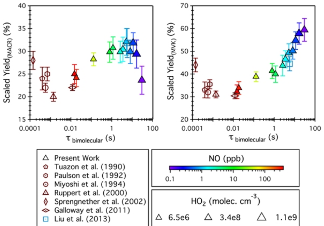
图1：异戊二烯的两个主要一代产物（异丁烯醛和甲基乙烯基酮）的产率在低浓度到高浓度氮氧化物条件下的变化。
