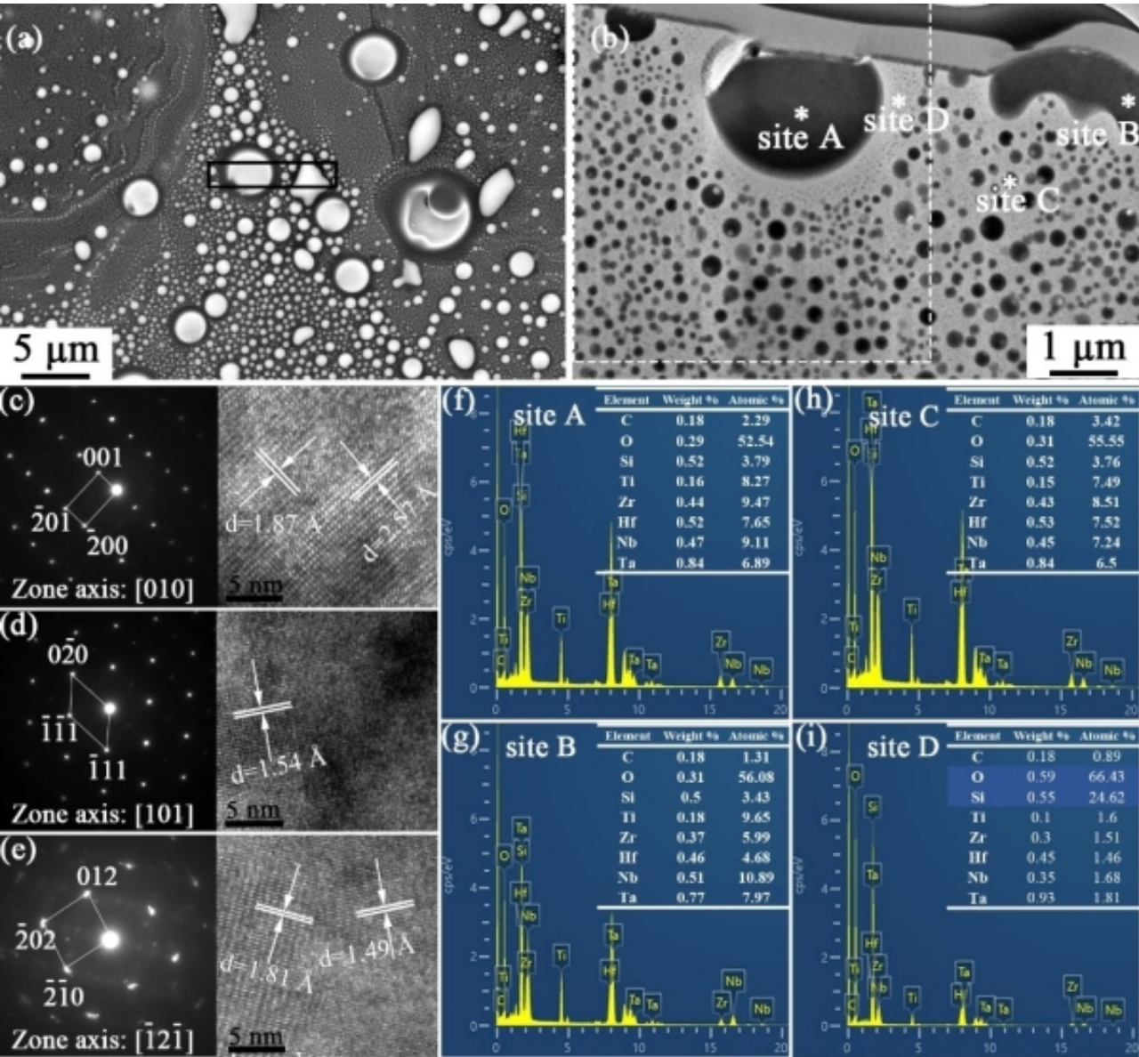
烧蚀中心形成的 (\text{TiZrHfNbTa})\text{O}_x ：微观形貌 (a、b)、晶体结构解析 (c-e) 及元素组成分析 (f-i)
