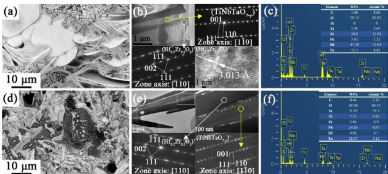
烧蚀表面片状 (\text{Hf}_{0.5}\text{Zr}_{0.5}\text{O}_2)' 和 (\text{TiNbTaO}_{7-y})' 纳米晶形成的“三明治”结构：微观形貌 (a、d)、晶体结构解析 (b、e) 及元素组成分析 (c、f)
