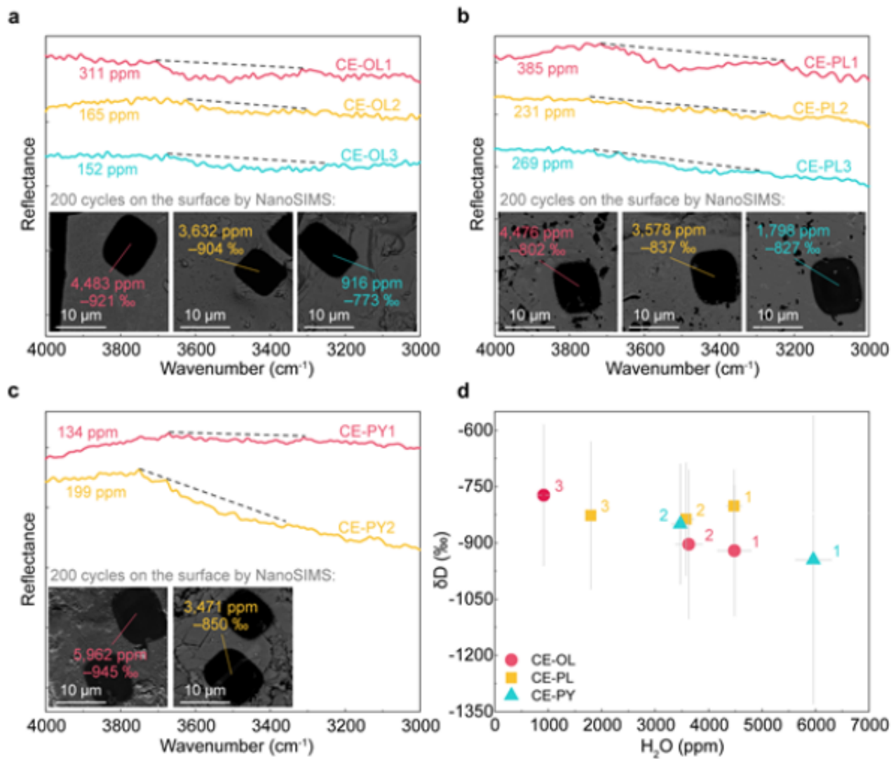
图1.矿物水含量和氢同位素比值
