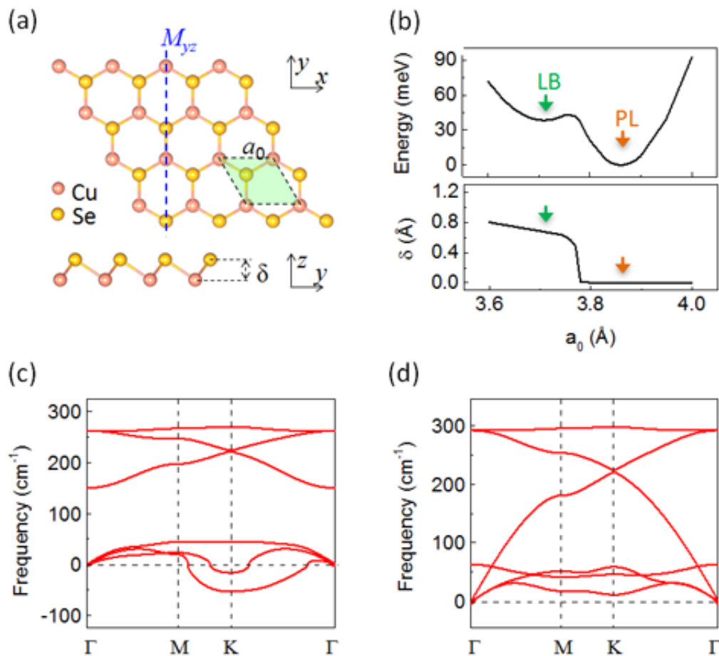
图1.单层硒化铜的原子结构和稳定性。
