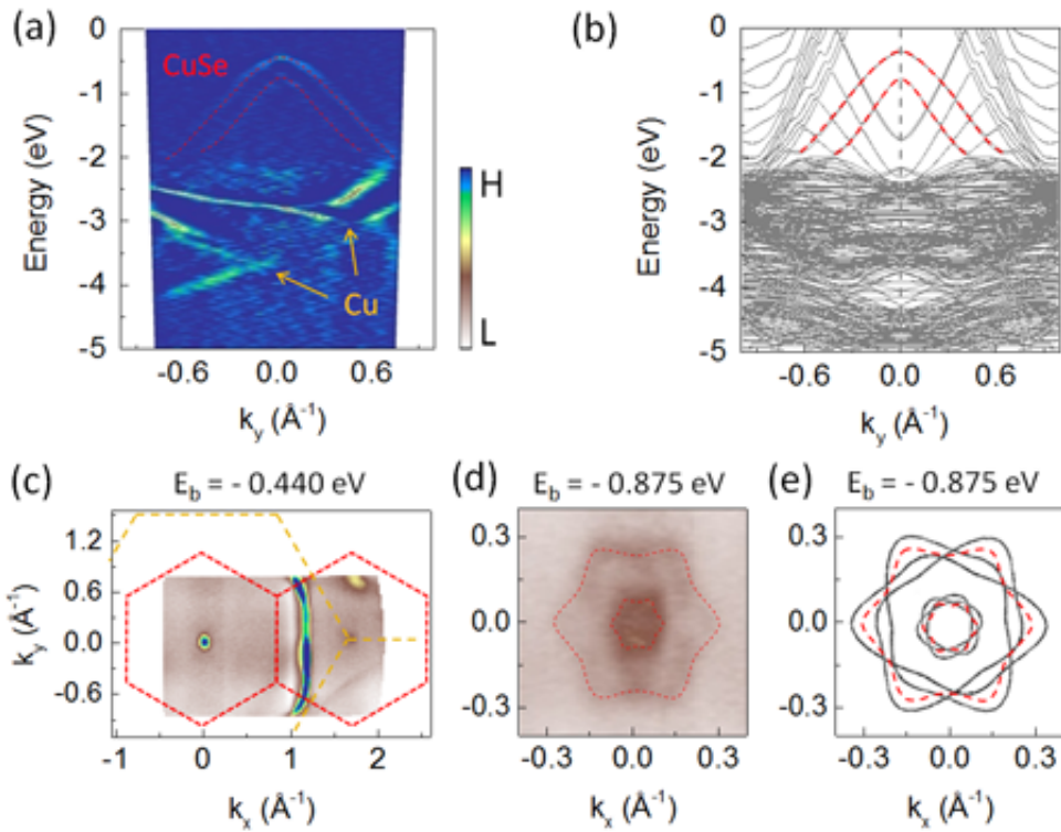
图4. 单层硒化铜在Cu(111)上的ARPES结果和第一性原理计算结果的对比图。
