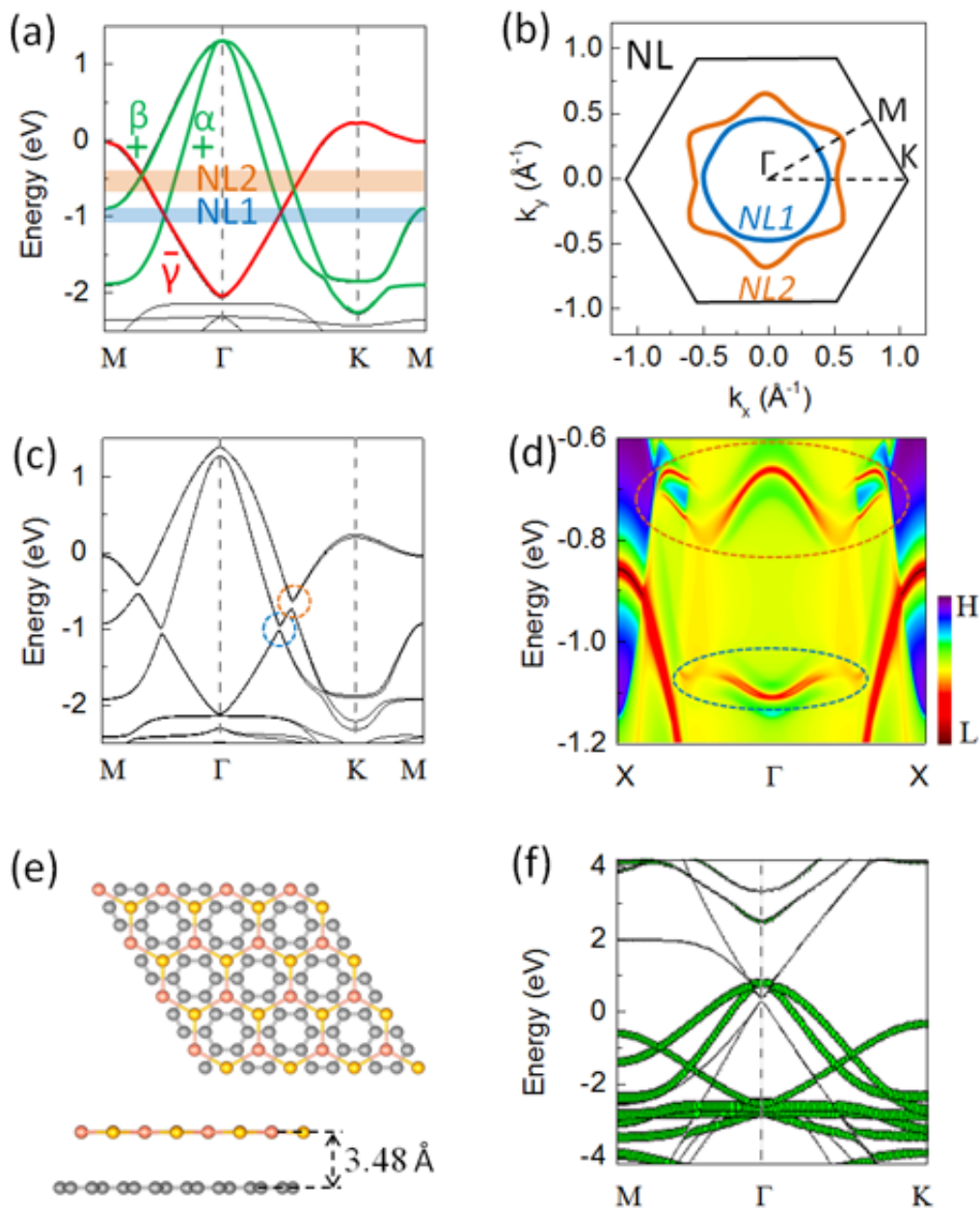
图2.单层硒化铜的电子结构和拓扑边界态，以及单层硒化铜在石墨烯上的原子结构和电子结构。
