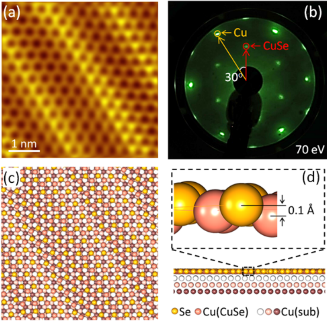
图3. 单层硒化铜在Cu(111)上的STM、LEED和原子结构图。
