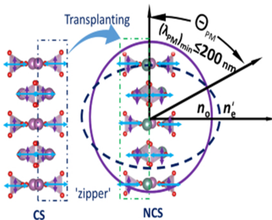
图：从中心化合中移植功能模块到非心化合物中设计新型深紫外非线性光学晶体
