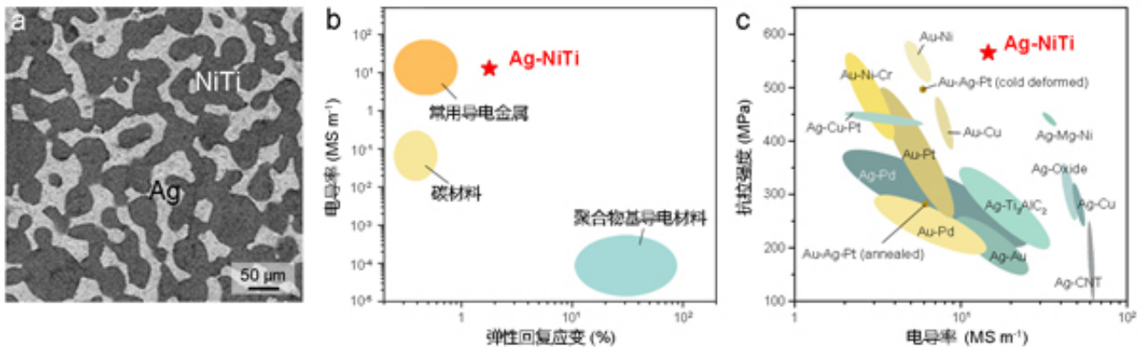
高弹性银-镍钛电接触材料的微观三维互穿结构及其性能与现有材料的比较
