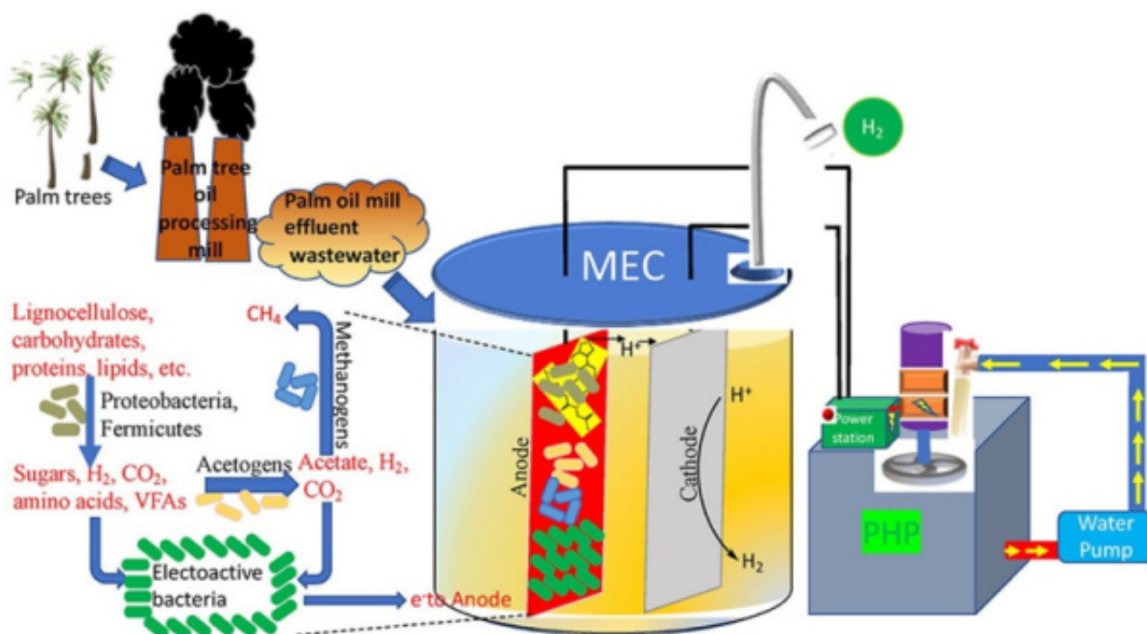
实验装置示意图
