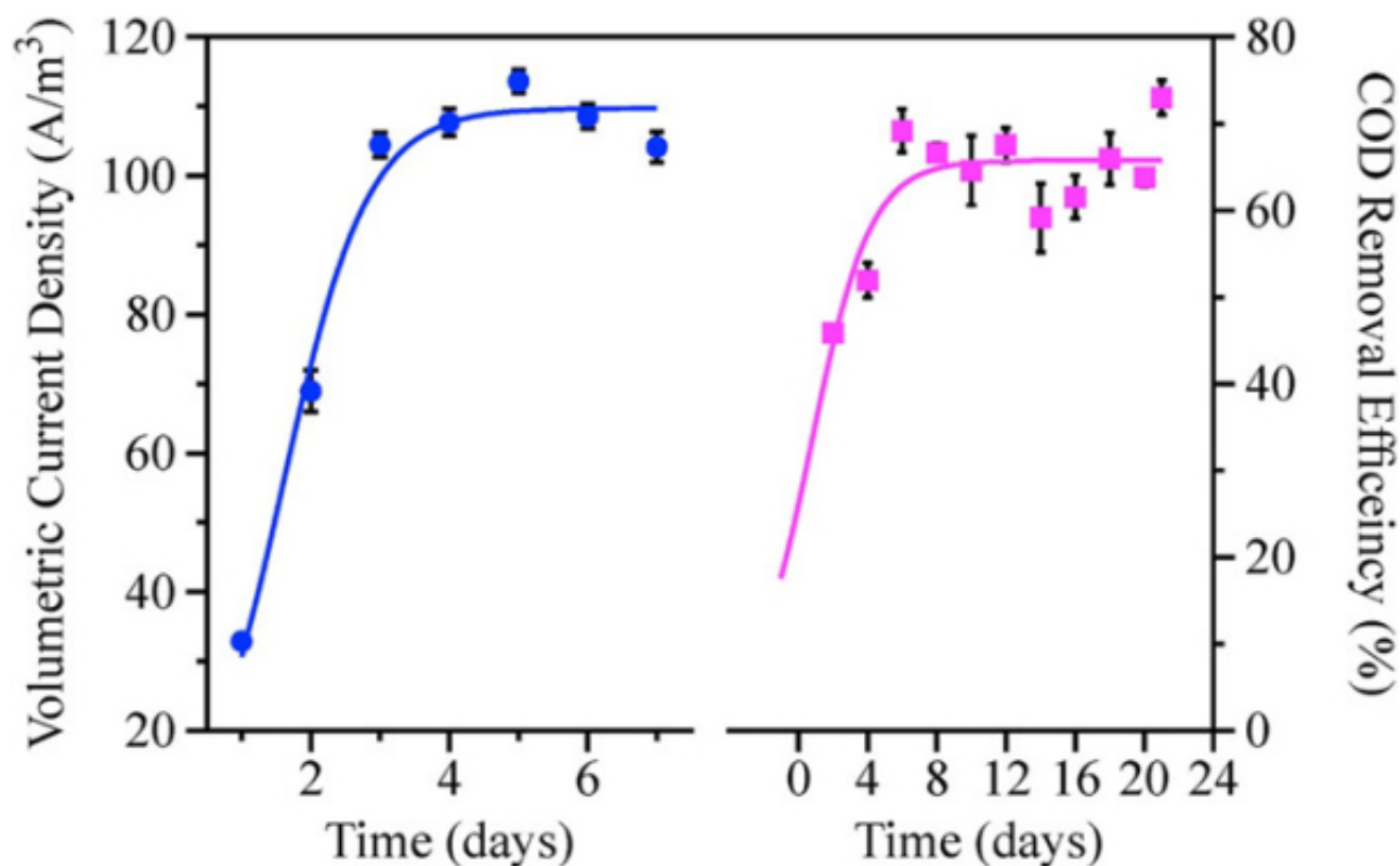
PHP-MEC反应器的关键性能指标（电流密度和COD去除率）随时间的变化
