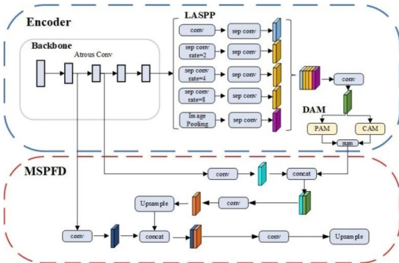
纳米颗粒分割模块结构示意图
