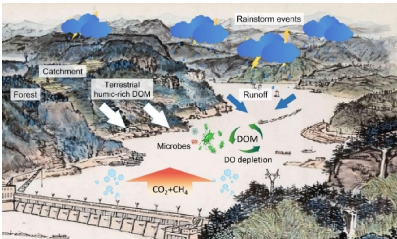
图1.暴雨事件促进陆源DOM输入及碳排放机制图
