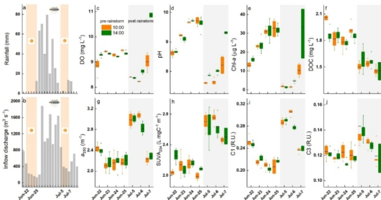
图2.暴雨前后新安江上游流域降雨量及来水量，溶解氧、pH、叶绿素a、溶解性有机碳DOC、DOM光谱吸收、紫外比吸收系数、陆源组分的高频变化特征
