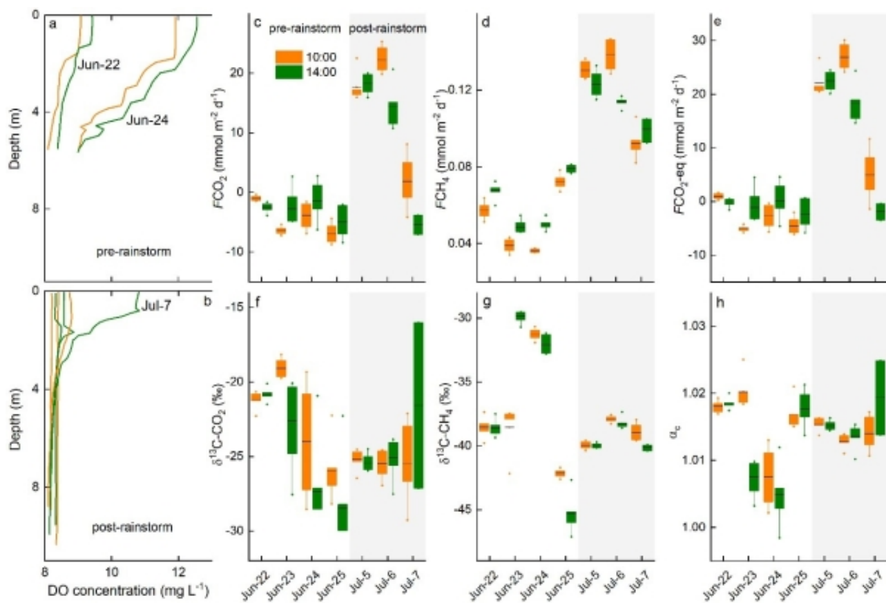
图3.暴雨前后街口站溶解氧垂向剖面变化特征以及二氧化碳、甲烷的排放通量与同位素组成的高频变化特征
