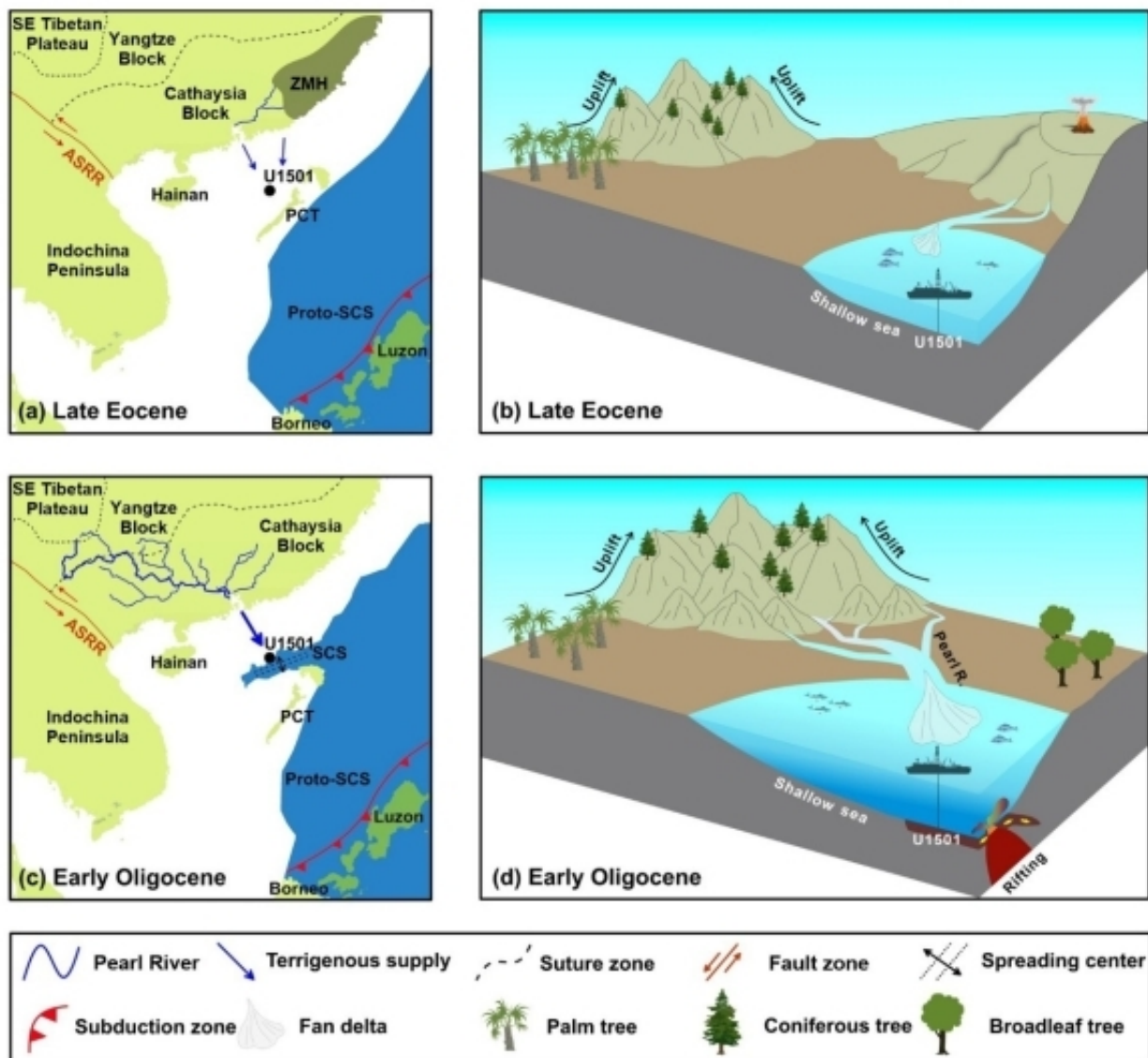
图4.晚始新世以来珠江演化示意图
