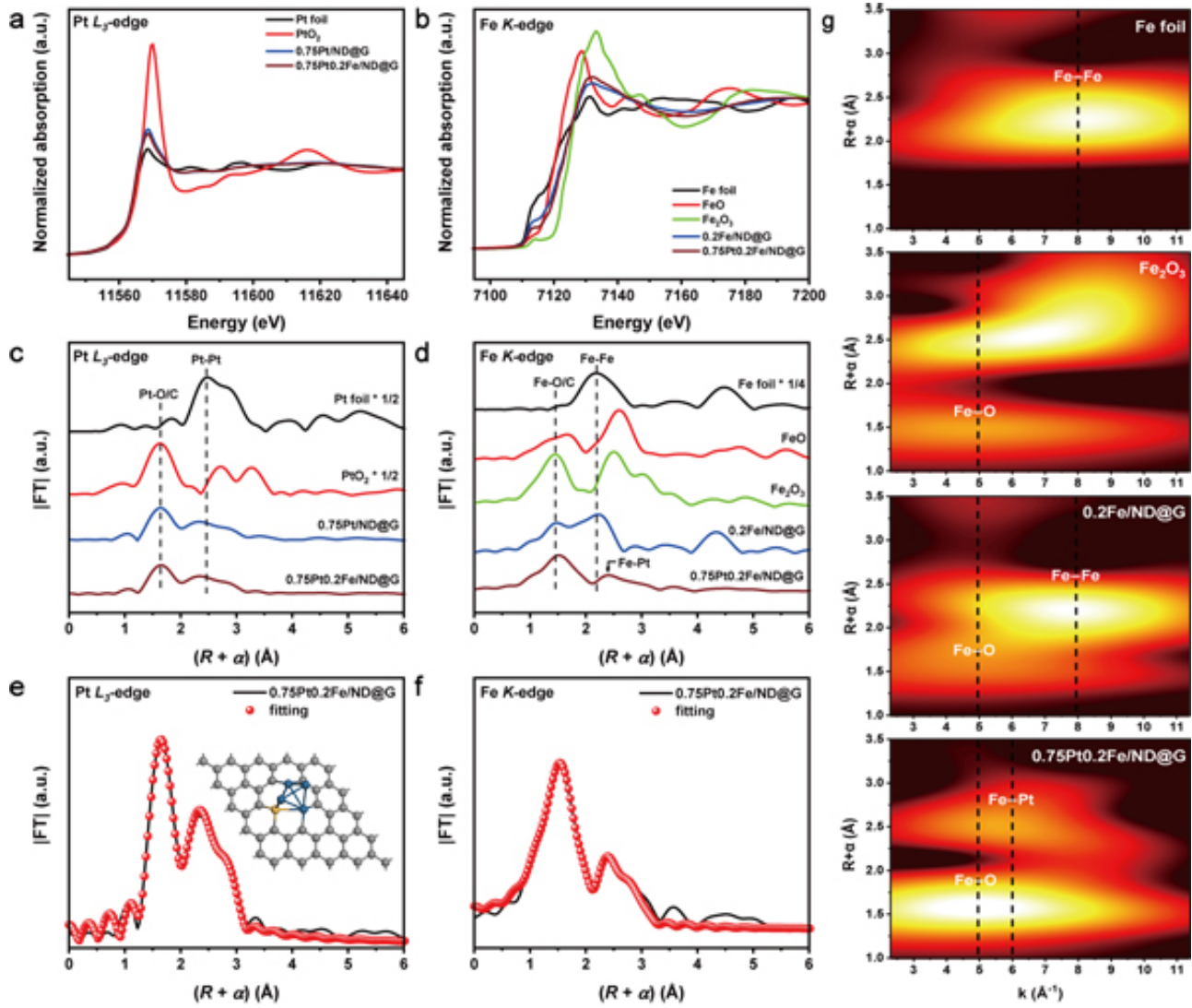
图2.全暴露PtFe双金属团簇 ( 0.75\text{Pt}0.2\text{Fe}/\text{ND}@G ) 的XAFS表征
