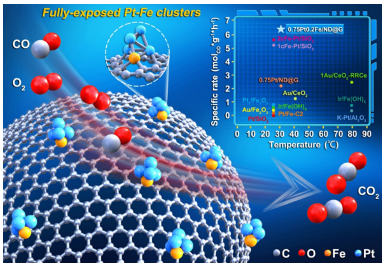
图4.亚纳米全暴露PtFe团簇催化CO选择性氧化示意图
