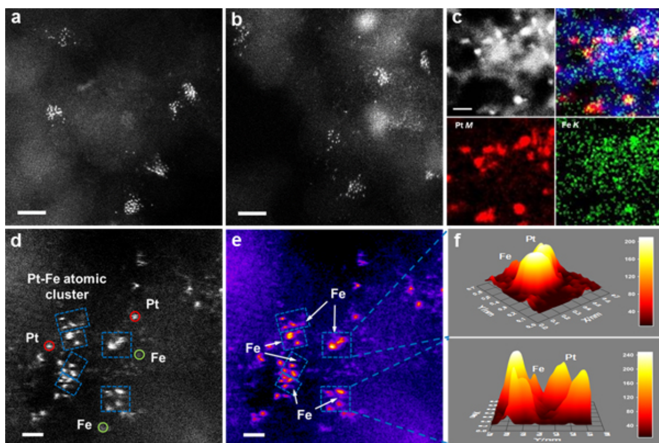
图1.全暴露PtFe双金属团簇（0.75Pt0.2Fe/ND@G）的HAADF-STEM表征
