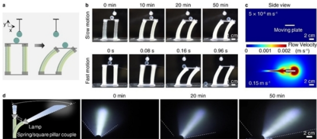
图2.仿松塔结构的超慢驱动装置
