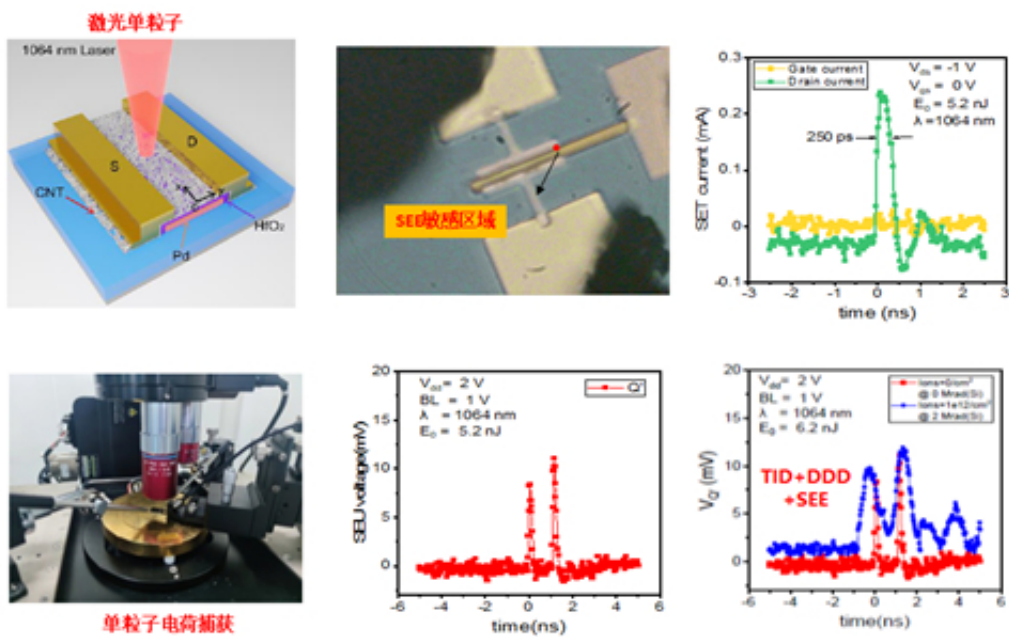
图3 碳纳米管电子器件单粒子效应响应特征
