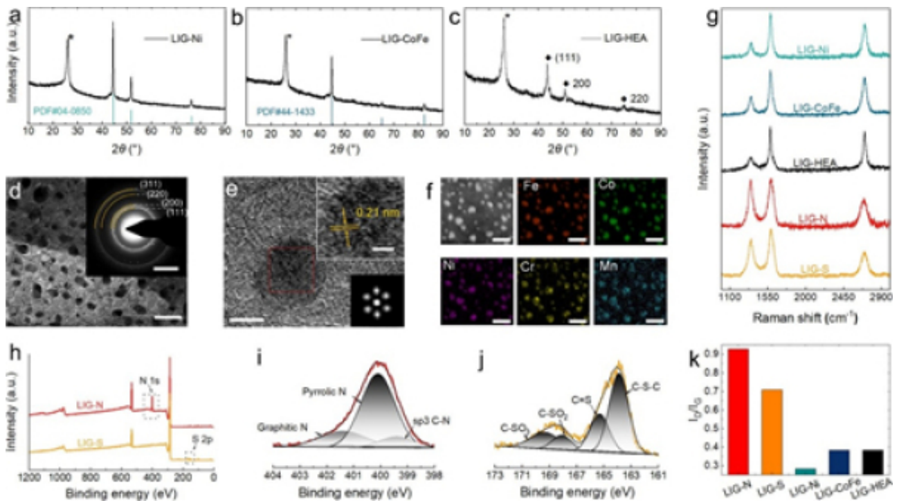
图2.三维石墨烯功能复合材料的制备表征
