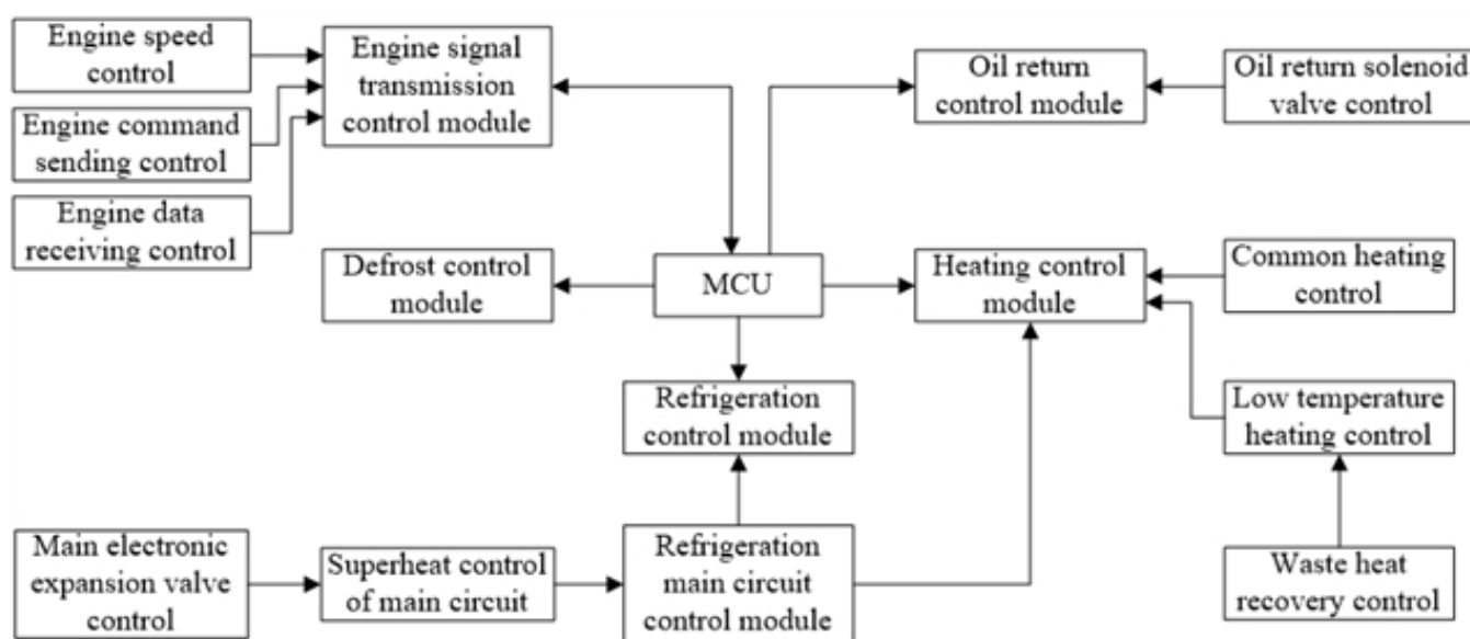
GHP主控制器主要功能模块
