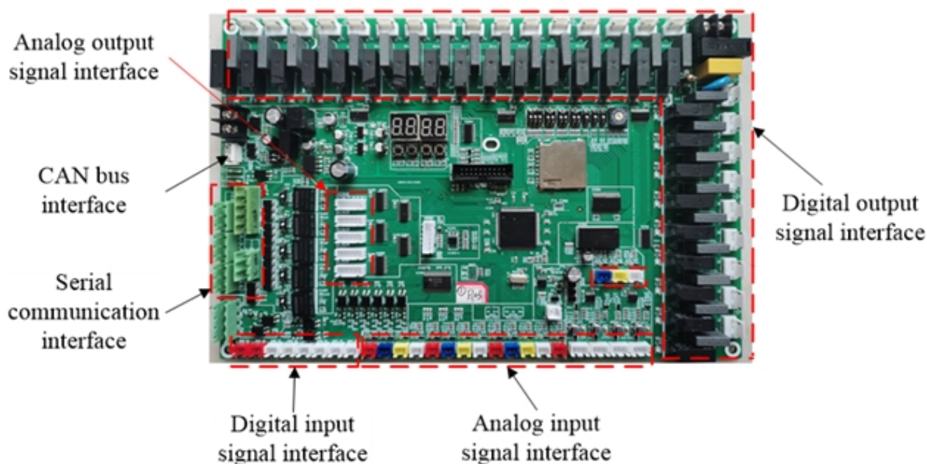
GHP主控制器电路板
