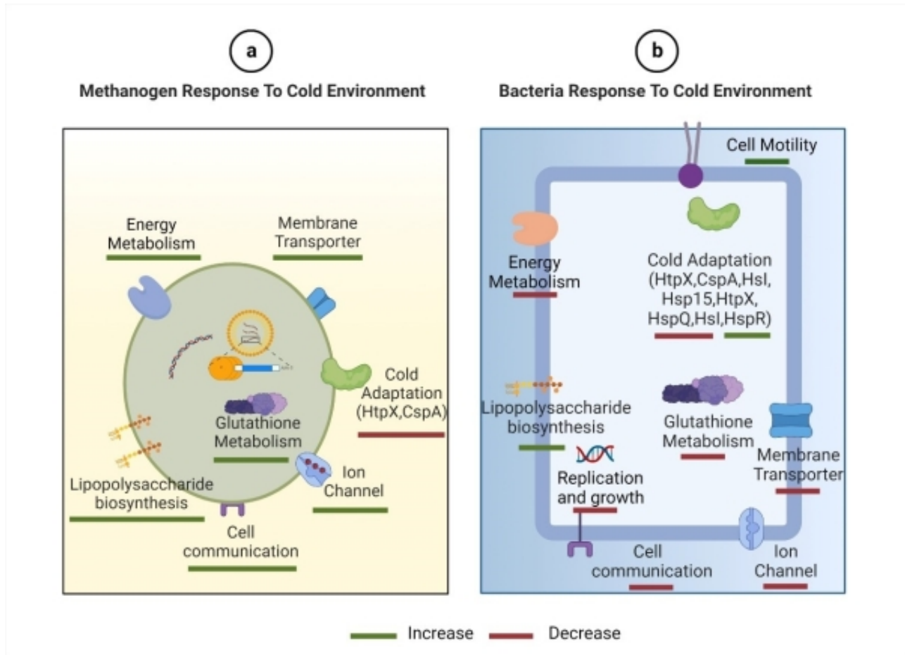
图1.低温对厌氧消化微生物代谢的影响。a、产甲烷菌;b、细菌。
