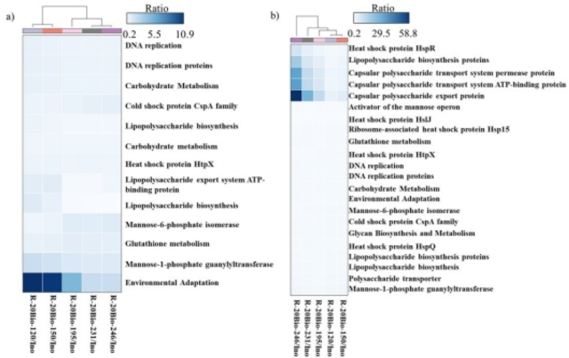
图3.生物强化对微生物基因丰度的影响。a)古菌;b)细菌(Ino：接种物)。
